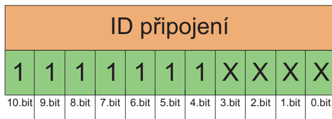
Obr. 1.20: Identifikátor CAN - neplatný rozsah.
