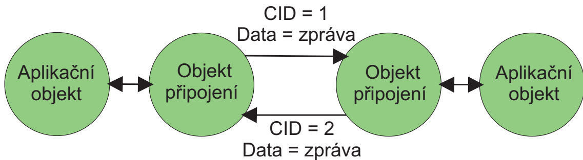
Obr. 1.4: Komunikace objektů.
