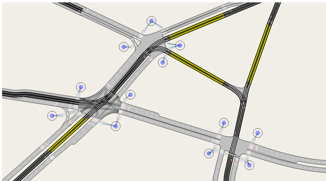
Obrázek 4.3: Uspořádání varianty 3
