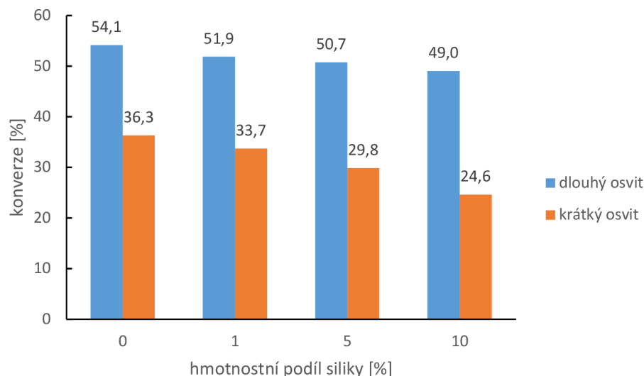
Obrázek 39 Sloupcový graf pro porovnání stupně konverze v závislosti na přidavku siliky do systému UDMA/TEGDMA – krátký osvit
