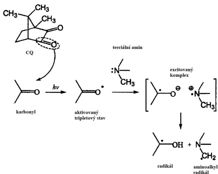
Obrázek 9 Schéma vzniku radikálů pomocí kafarchinonu a terciálního aminu [6]
