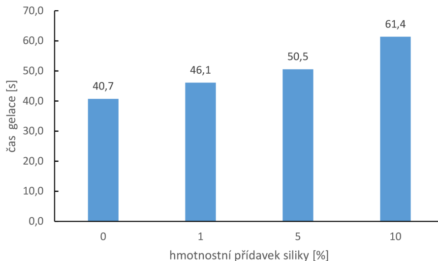
Obrázek 41 Sloupkový graf pro znázornění výsledných časů bodu gelace systému UTS
