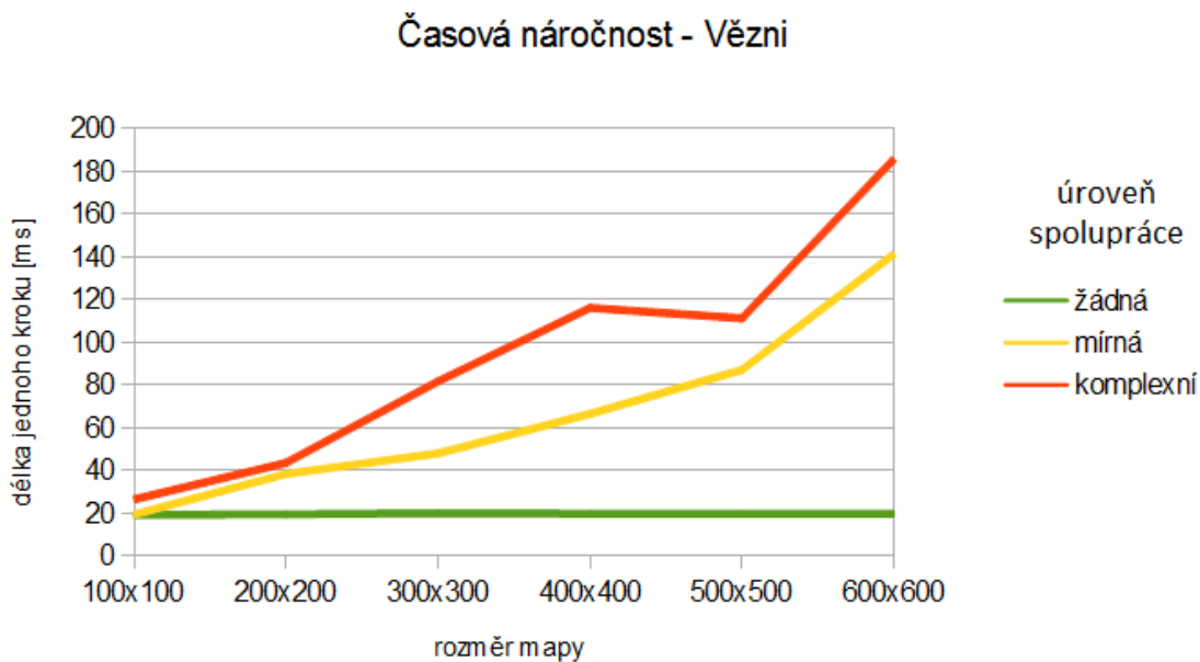
Obrázek 7.3: Časová náročnost rozhodování vězňů v závislosti na velikosti mapy.
