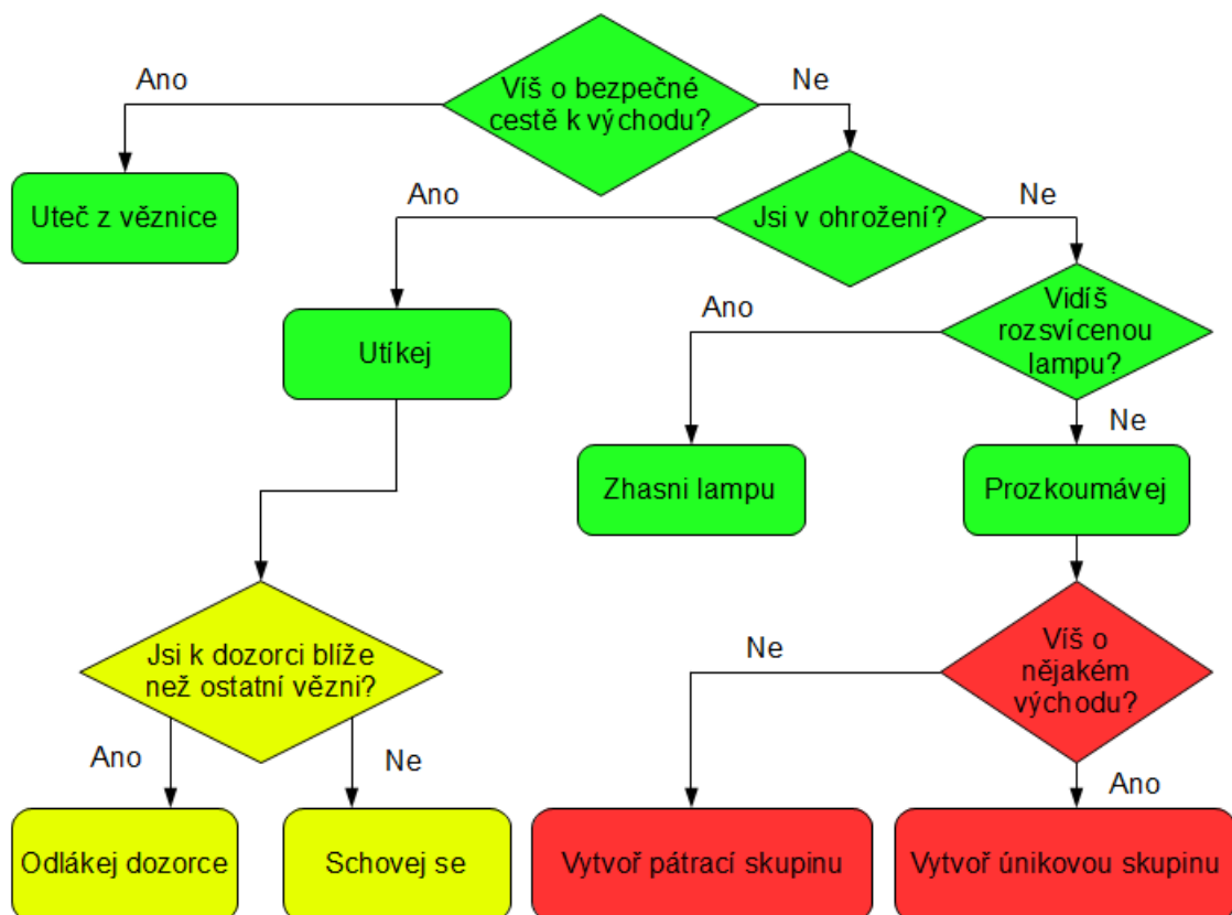
Obrázek 5.1: Rozhodovací strom vězně.
