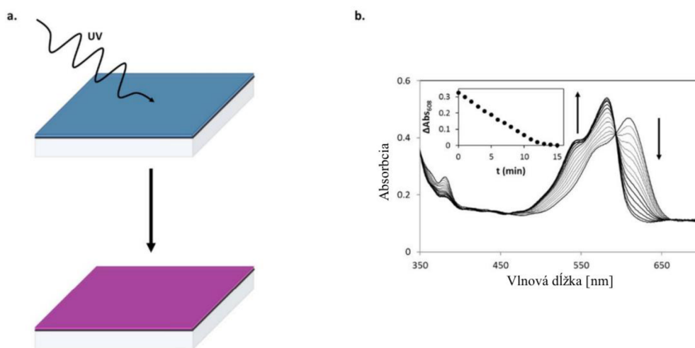
Obr. 10: (a.) Schematické znázornenie systému ožarovania resazurinu, v ktorom sa vzorka pokrytá resazurinom po ožiarení UV žiarením zmení z modrej na ružovú a (b.) typický súbor spektrálnych zmien UV/Vis, ktoré vznikli pri teste resazurinu, s vloženým diagramom zobrazujúcim profil rozpadu pri 608 nm. 30
