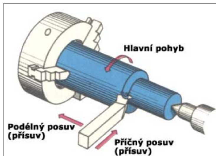
Obrázek 14: Princip soustružení (Zdroj: www.osu.cz )
