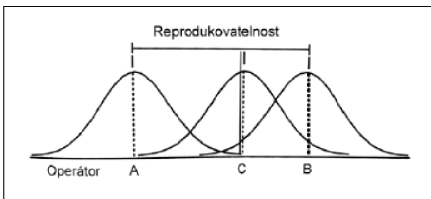
Obrázek 13: Reprodukovatelnost měření (Zdroj: Česká společnost pro jakost, 2011)
