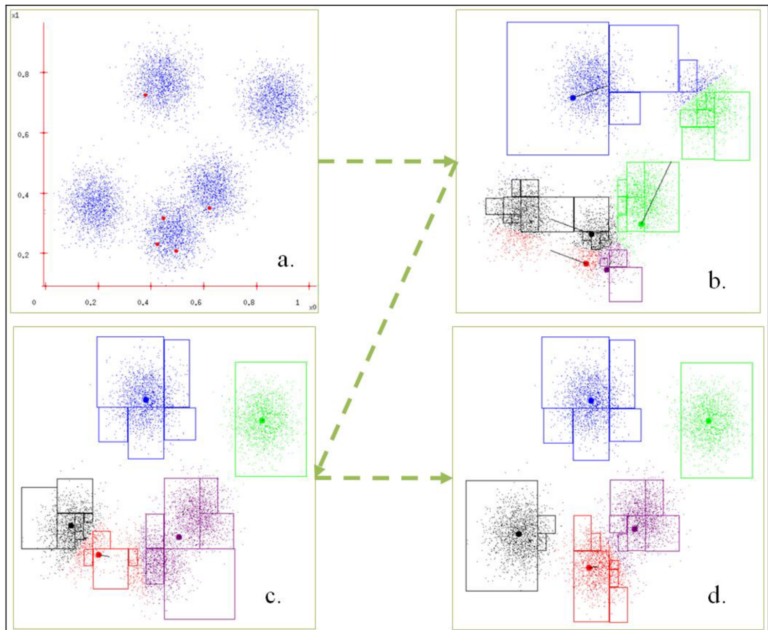
Obrázek 4.6: Názorné předvedení algoritmu pomocí obrázků: a) umístění k vzorků do prostoru. b) + c) přiřazování bodů do jednotlivých středů d) konečné rozpození shluků a k nim přiřazených bodů [6]
