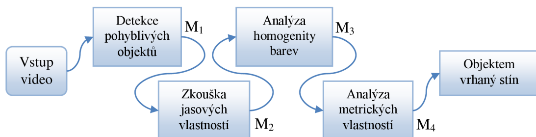
Obrázek 4.12: Blokové schéma algoritmu pro detekci stínů
