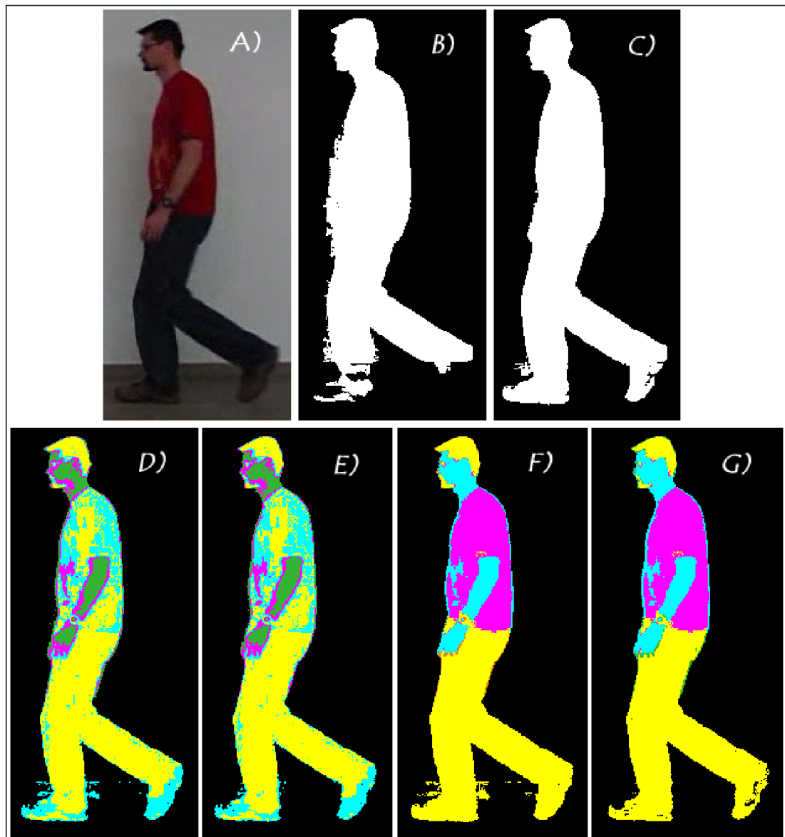
Obrázek 5.12: Porovnání výsledků segmentace na jednom z obrázků různými metodami: A) původní obrázek, B) rozdílové snímky, C) rozdílové snímky s transformací jasové stupnice, D) metoda k-mean s transformace jasové stupnice, E) metoda k-mean s transformace jasové stupnice a detekcí stínů, F) metoda mean shift s transformace jasové stupnice, G) metoda mean shift s transformace jasové stupnice a detekcí stínů
