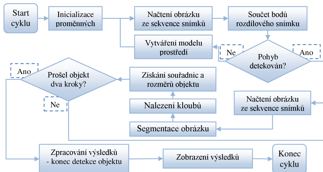
Obrázek 5.2: Blokové schéma hlavního cyklu programu
