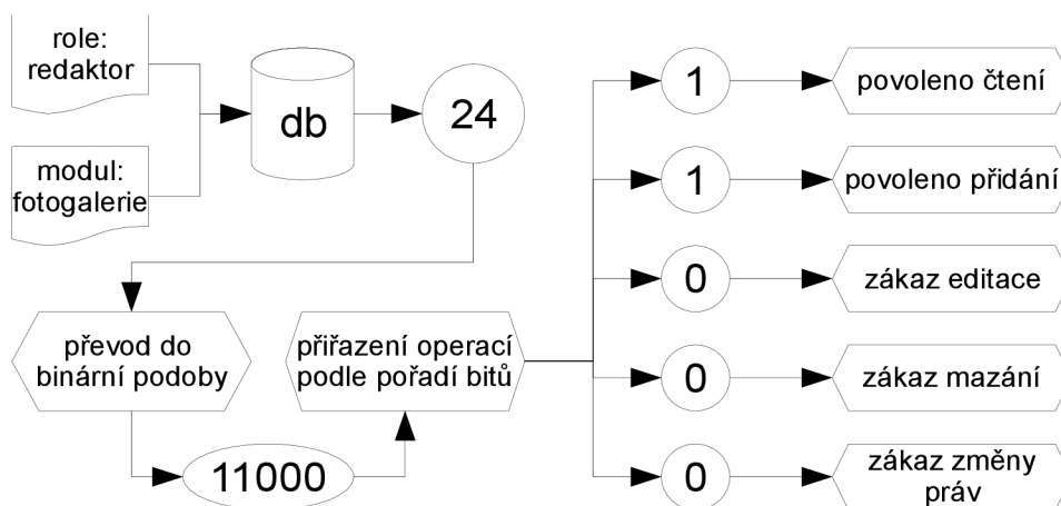
Obrázek 4.12: Načítání a zpracování přístupových dat z databáze
