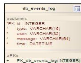
Obrázek 4.7: Tabulka záznamů událostí (UML)
