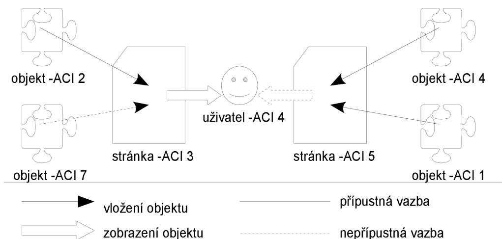
Obrázek 3.11: Schéma řízení přístupu k objektům
