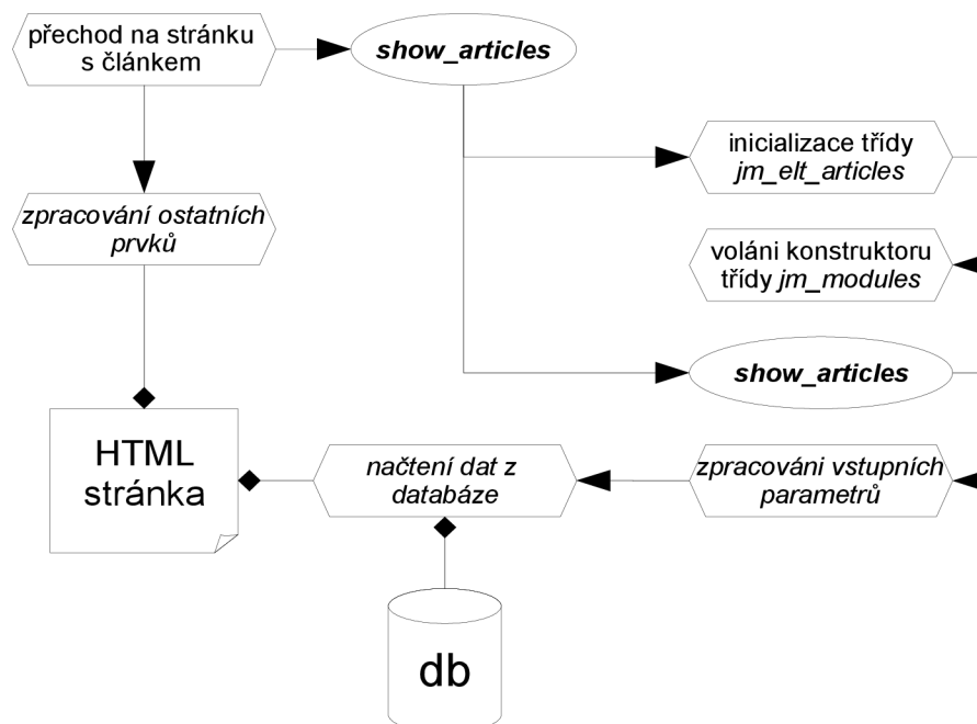
Obrázek 4.16: Práce se články
