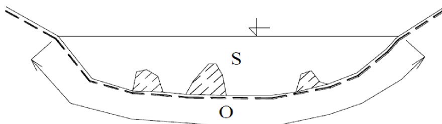
Obrázek 4.2 Řez koryta, určení základních charakteristik profilu se zobrazením makrodrsnotí
