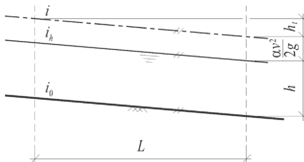
Obrázek 4.1 Ustálené proudění
