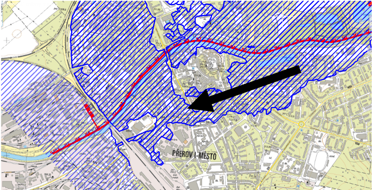
Obrázek 7.2 Ukázka rozlivu s vyznačeným směrem proudění
