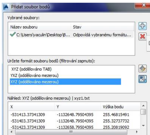
Obrázek 6.3 Přidání souboru bodů do DMT
