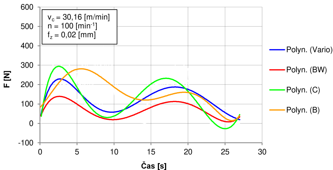
Obr. 5.22 Řezání při řezných podmínkách dle katalogu bez vlivu odpružení.
