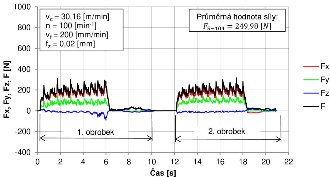
Obr. 5.10 Řez bez vlivu odpružení pilovým kotoučem s ozubením C při řezných podmínkách č. 1.
