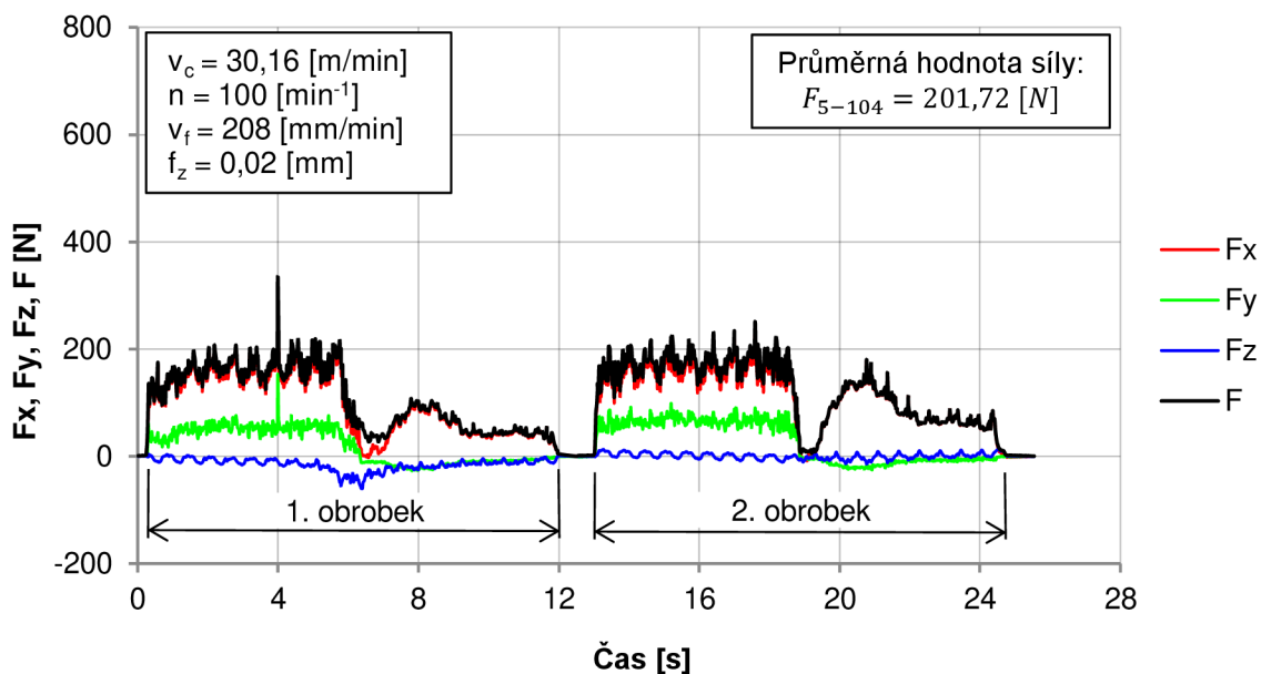
Obr. 5.18 Řez bez vlivu odpružení pilovým kotoučem s ozubením VARIO B při řezných podmínkách č. 3.
