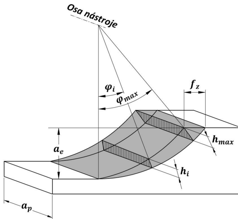
Obr. 1.6 Znárodnění průřezu třísky – podle [12].
