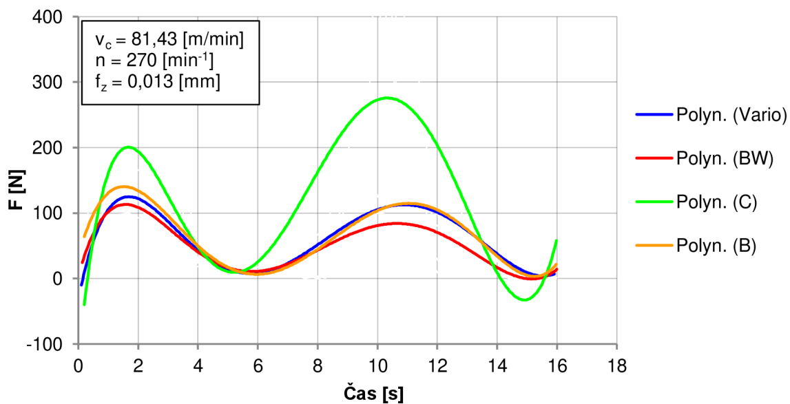
Obr. 5.25 Řezání při řezných podmínkách dle Fischer Vyškov, spol. s r. o., s vlivem odpružení.
