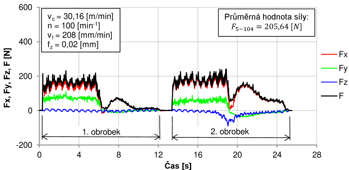
Obr. 5.19 Řez s vlivem odpružení pilovým kotoučem s ozubením VARIO B při řezných podmínkách č. 3.
