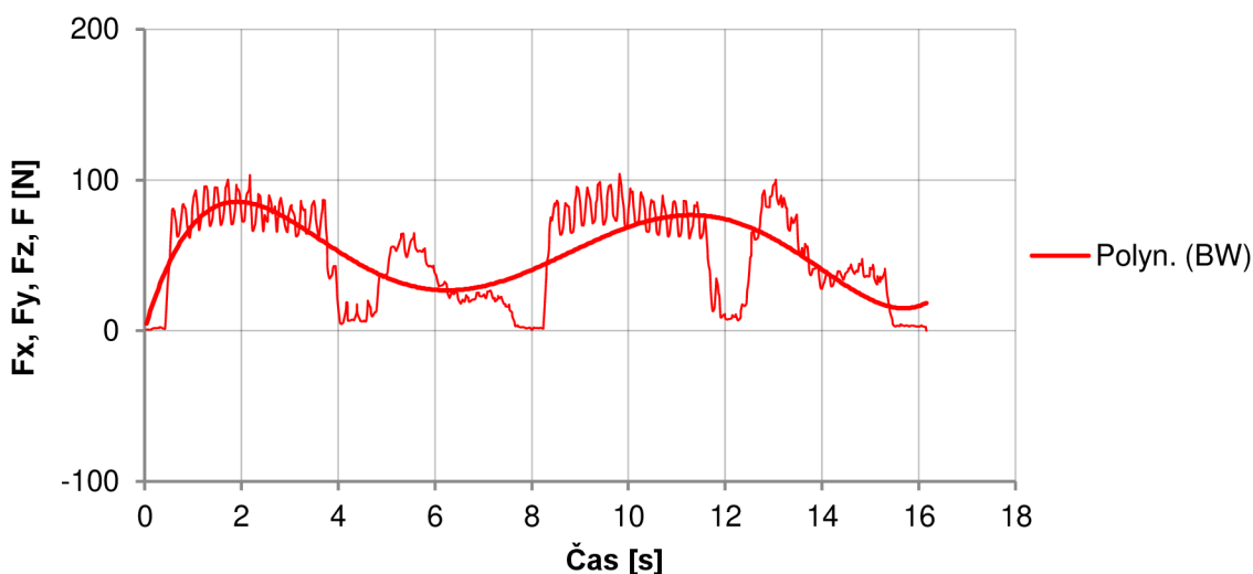
Obr. 5.5 Ukázka proložení výslednice sil polynomem šestého stupně.
