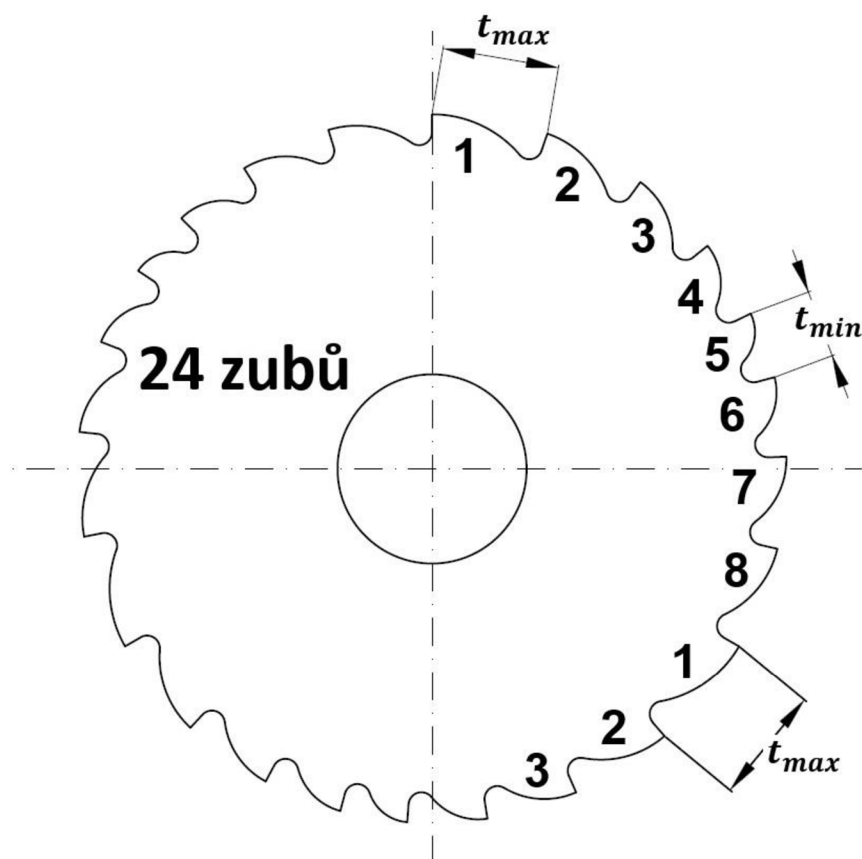
Obr. 2.11 Ozubení VARIO B (V8) – podle [19,20].
