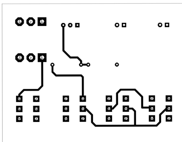
Obr. 9-20 Med' - vrstva Bottom
