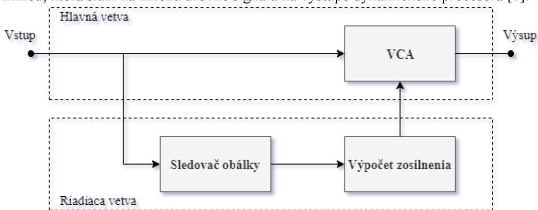
Obr. 1-1 Bloková schéma dynamického procesoru
