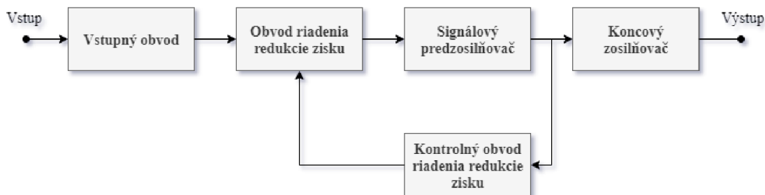
Obr. 6-1 Bloková schéma kompresora 1176
