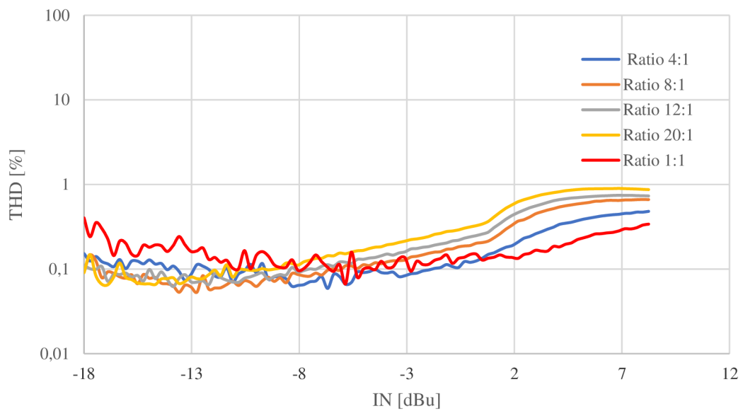
Obr. 9-4 THD kompresora 1176
