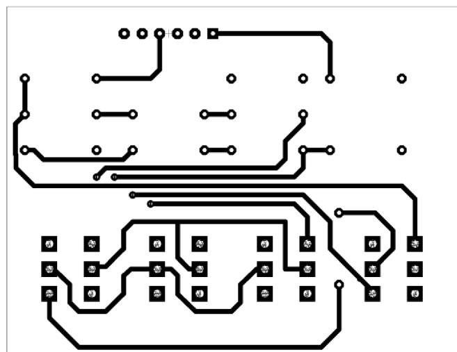
Obr. 9-15 Med' - vrstva Bottom
