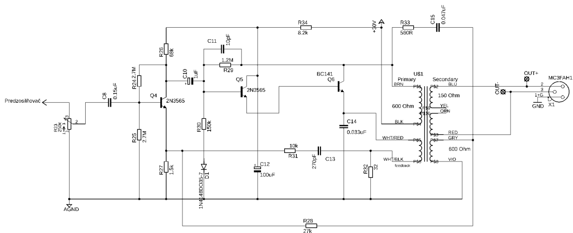
Obr. 6-6 Schéma obvodu koncového zosilňovača
