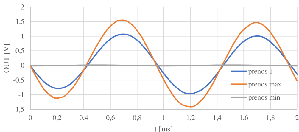
Obr. 6-2 Časová analýza vstupného obvodu
