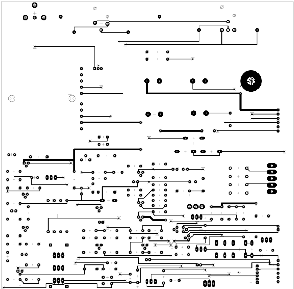
Obr. 9-11 Med 3 - vrstva Bottom
