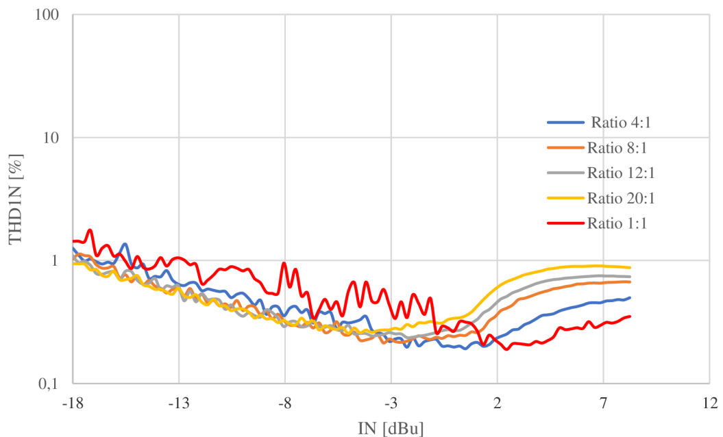
Obr. 9-5 THD+N kompresora 1176
