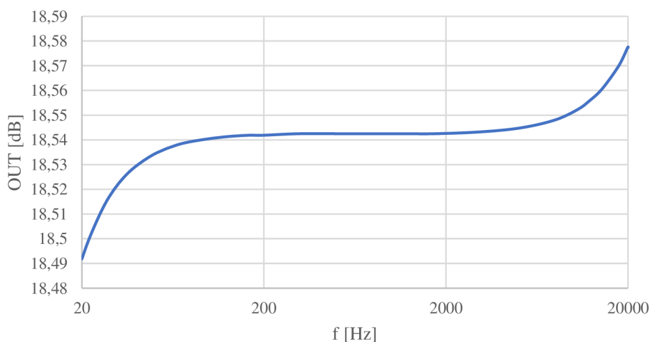
Obr. 6-9 Frekvenčná odozva Kontrolného obvodu riadenia redukcie zisku
