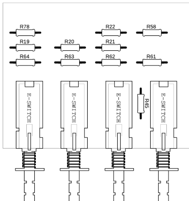
Obr. 9-16 Osadenie súčiastok - vrstva Top
