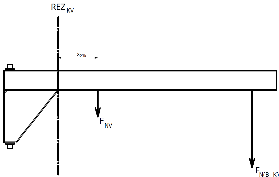
Obrázek 19 Zatížení výložníku
