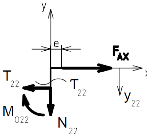
Obrázek 9 Řešení VVÚ v intervalu \tau_{22}
