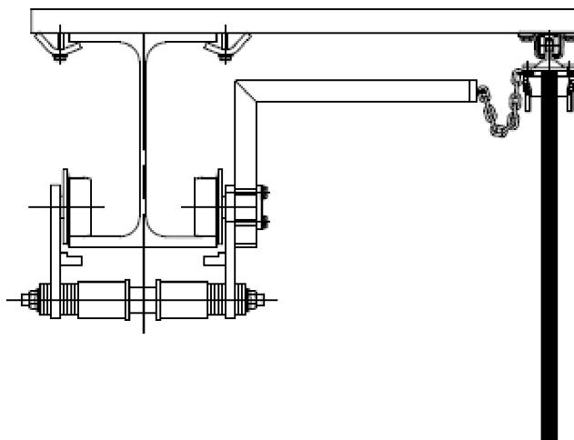
Obrázek 32 Unašeč vlečného kabelu Abus [3]
