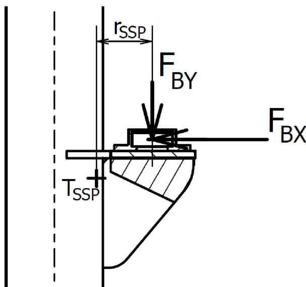
Obrázek 27 Návrhové zatížení spodní patky
