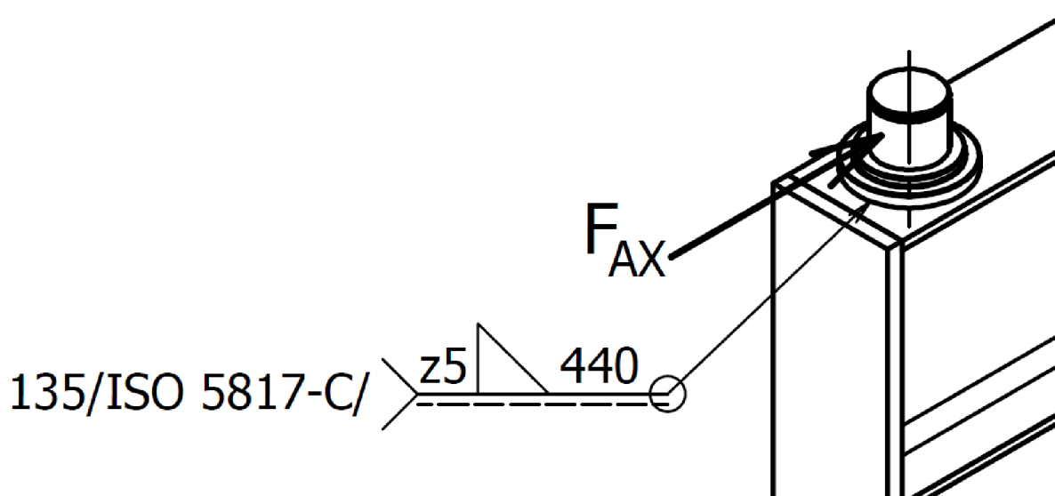
Obrázek 29 Zatížení čepů výložníku
