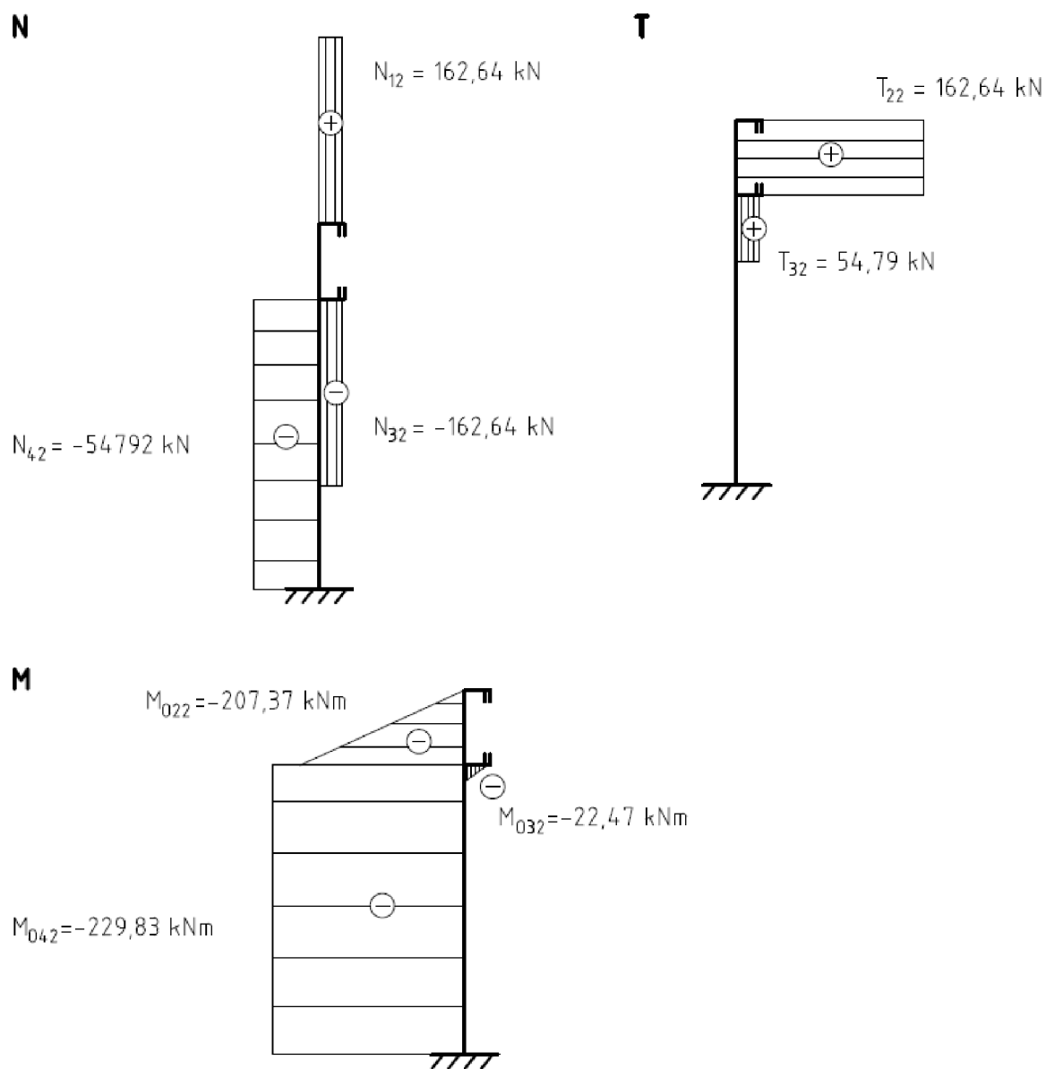
Obrázek 12 Výsledné VVÚ sloupu
