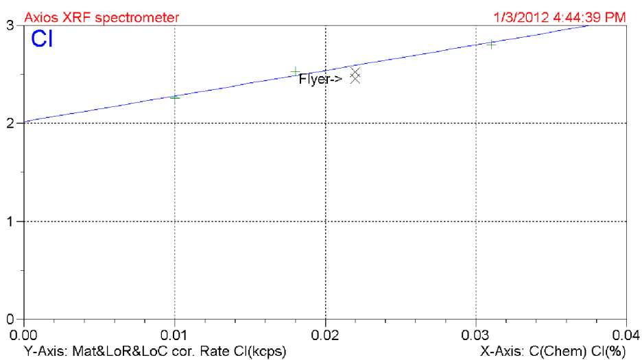
Obrázek 33 - Kalibrační křivka pro chlór
