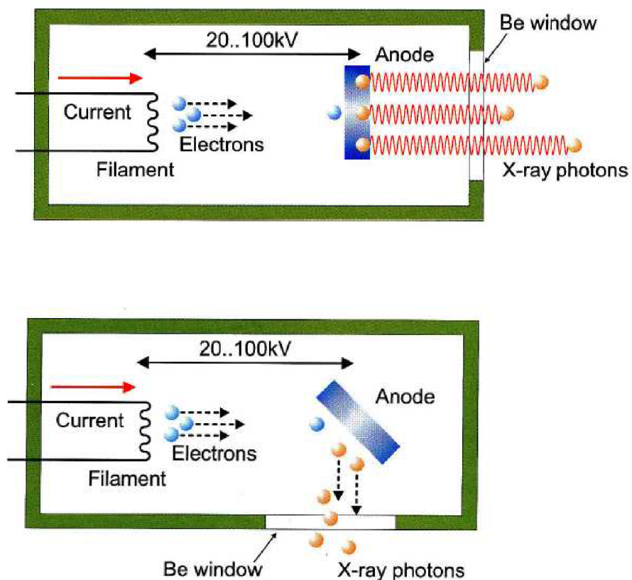
Obrázek 5 - Typy rentgenek - Transparentní s koncovým okénkem a reflexní s postranním okénkem [2]
