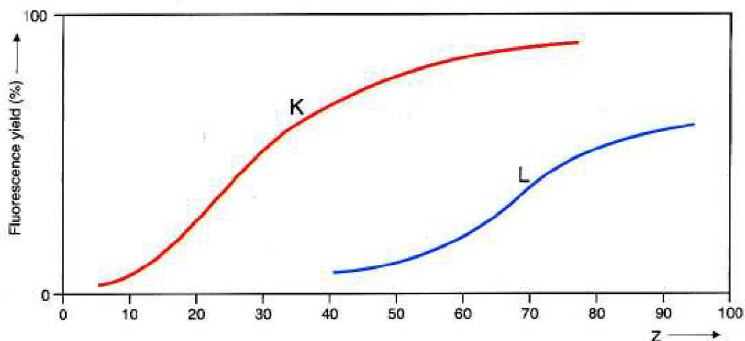
Obrázek 13 - Fluorescenční výtěžek [2]
