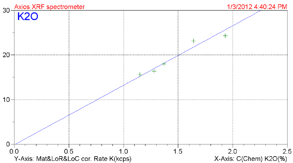
Obrázek 27 - Kalibrační křivka pro oxid draselný
