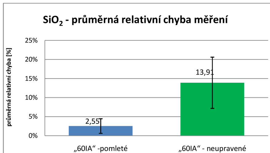
Graf 17 - SiO 2 - průměrná relativní chyba měření
