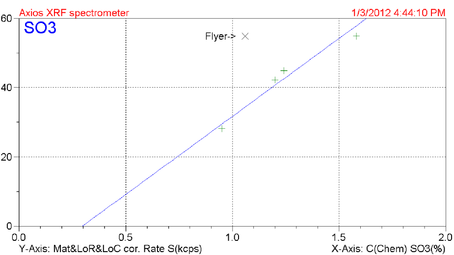
Obrázek 30 - Kalibrační křivka pro oxid sírový
