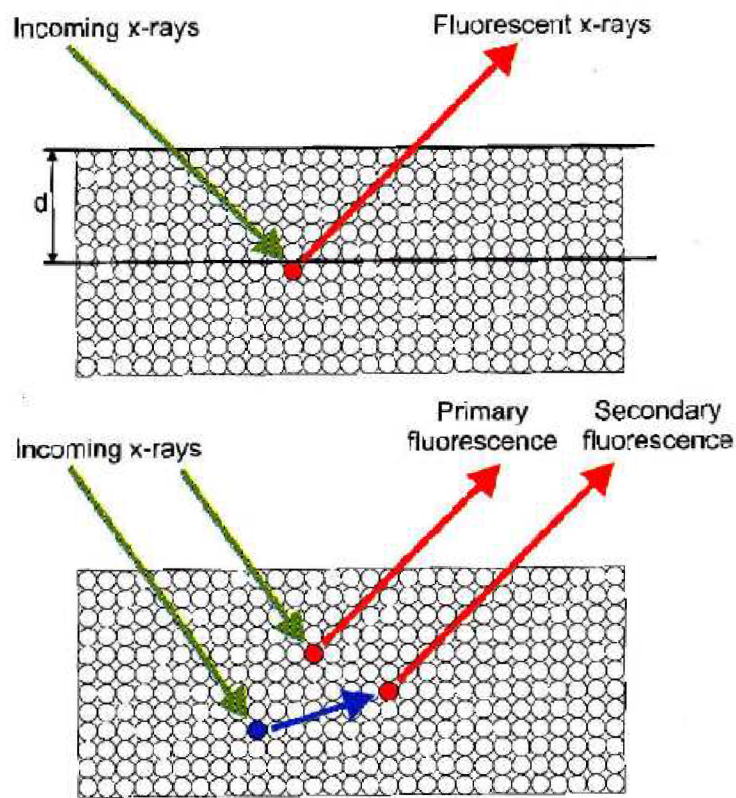
Obrázek 16 - Princip absorpce a přibuzování [2]
