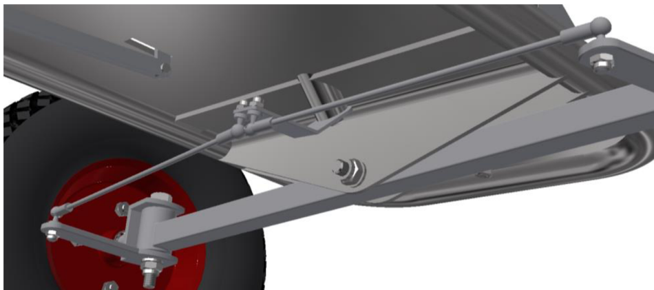
Obr. 4.20 Táhla řízení
