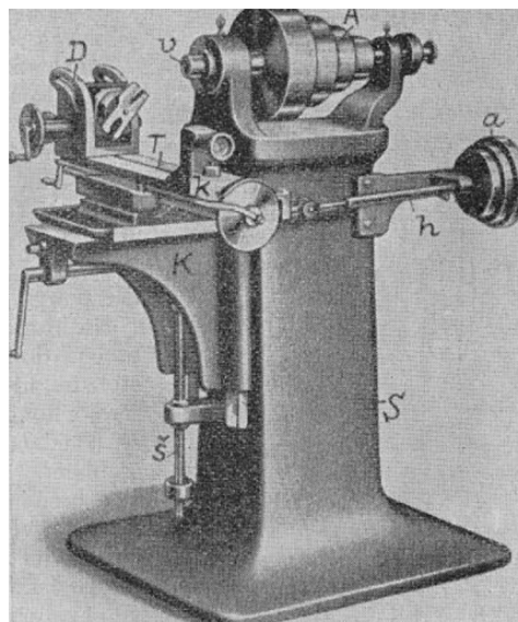
Obr. 1.3 Univerzální frézka z roku 1862 [17].
