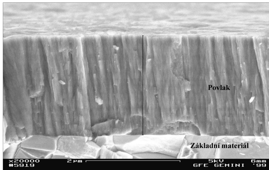
Obr. 3.8 Morfologie povlaku CC AluSpeed ® [3].
