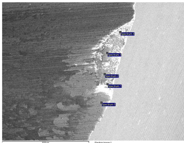
Obr. 4.5 Ukázka vylomené části břítu na jednom ze zubů čtyřbřité frézy s povlakem TiAlN [18].
