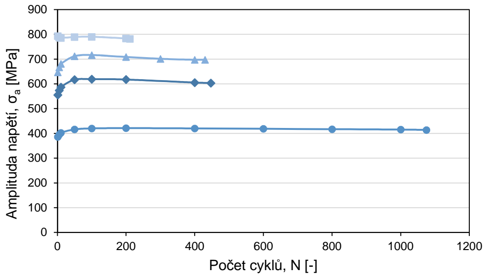
Obrázek 5.3: Křivky cyklického zpevnění a změkčení drátu NiTi při stejném předpětí a různých \epsilon_a v celém rozsahu životnosti.
