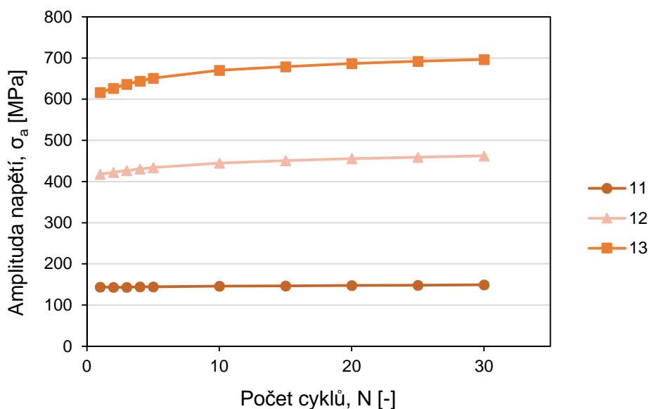
Obrázek 5.6: Křivky cyklického zpevnění drátu NiTi při stejném předpětí a různých \epsilon_a v prvních 30 cyklech.
