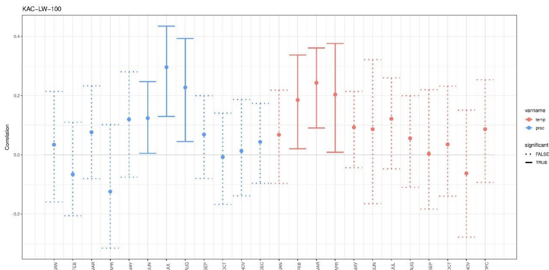
Obrázek 13 Korelace šířek letního dřeva s teplotou a úhrnem srážek, lokalita Kačkar
