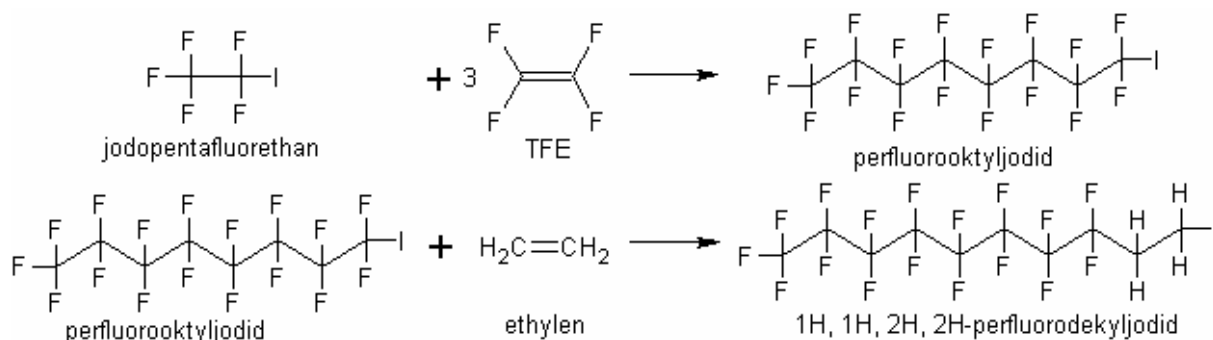
Obrázek 3 Příklad telomerace se třemi jednotkami TFE
