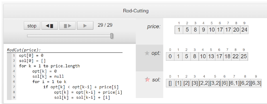
Obr. 3.4: Priebch riešenia úlohy Rezanie tyče . Pre vizualizáciu je využitá knižnica Vamonos . V ľavej časti sú ovládacie prvky a zdrojový kód, napravo tabuľky so vstupnými hodnotami, výsledkami optimálnych riešení podproblémov a aj tabuľka s celými riešeniami (prevzaté z [33]).
