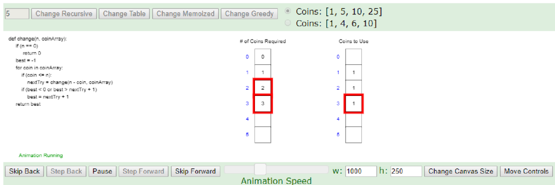
Obr. 3.3: Priebch riešenia úlohy Vydávanie mincí tabuľkovou metódou zdola-hore . Okrem dynamickej tabuľky je dostupný aj popis algoritmu. Rýchlosť animácie sa dá prispôsobiť, rovnako aj veľkosť plátna (prevzaté z [9]).
