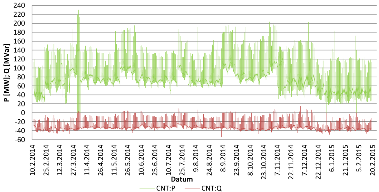
Obr. 6-1 Roční odběrový diagram P a Q transformátoru 400/110 kV v rozvodně CNT
