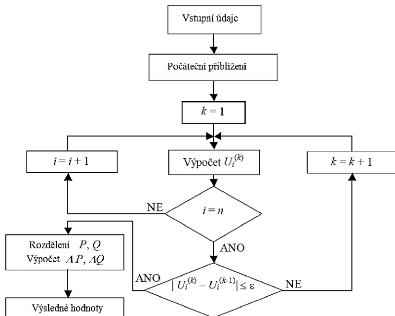
Obr. 4-5 Algoritmus řešení výpočtu Gauss – Seidlovou iterační metodou[6]
