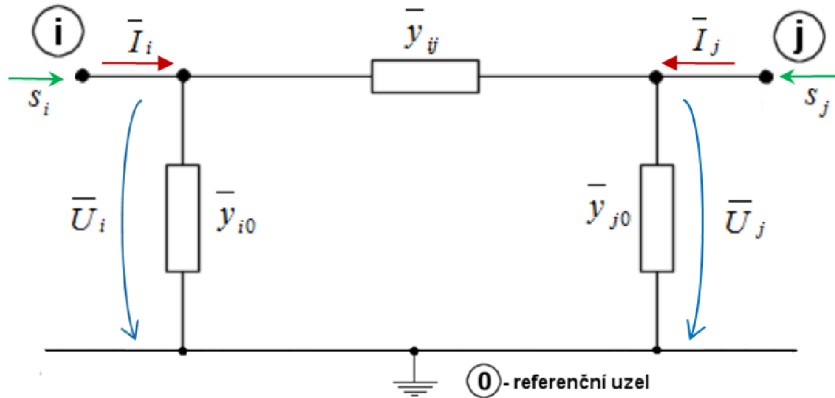
Obr. 4-4 Náhradní schéma \pi článku
