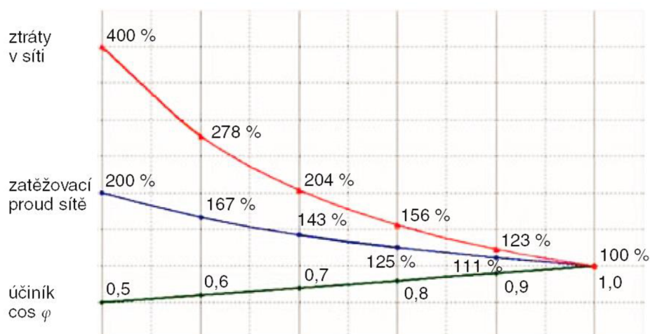
Obr. 3-2 Proudové zatížení (modře) a ztráty v síti (červeně) jako funkce účinníku (zeleně) [7]
