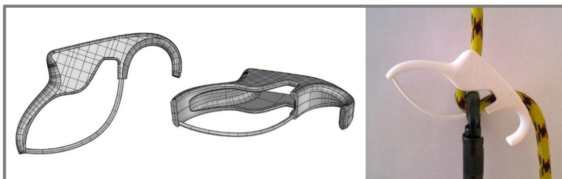
Obr. 4-19 Varianta C-IV
