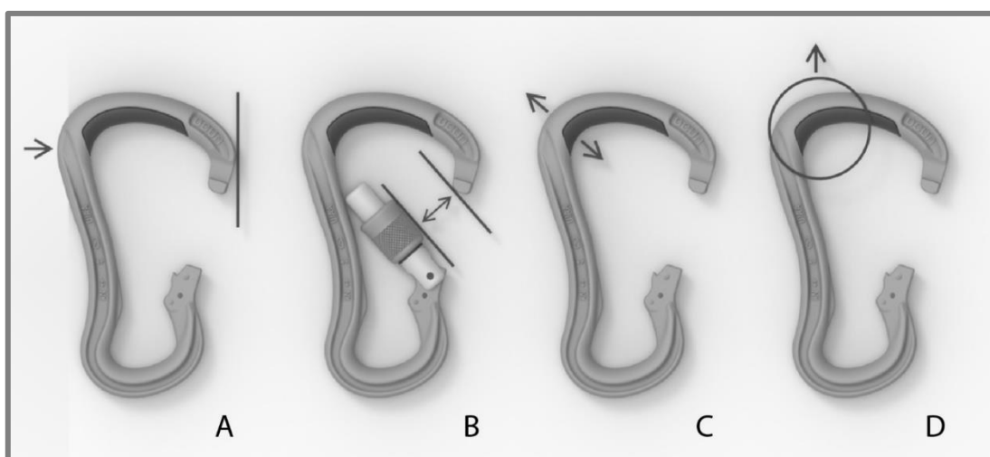
Obr. 5-4 Úpravy karabiny
