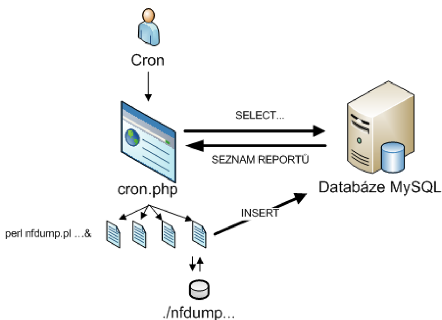
Obrázek 5 - Ilustrace načtení a zpracování dat z nástroje NfDump
