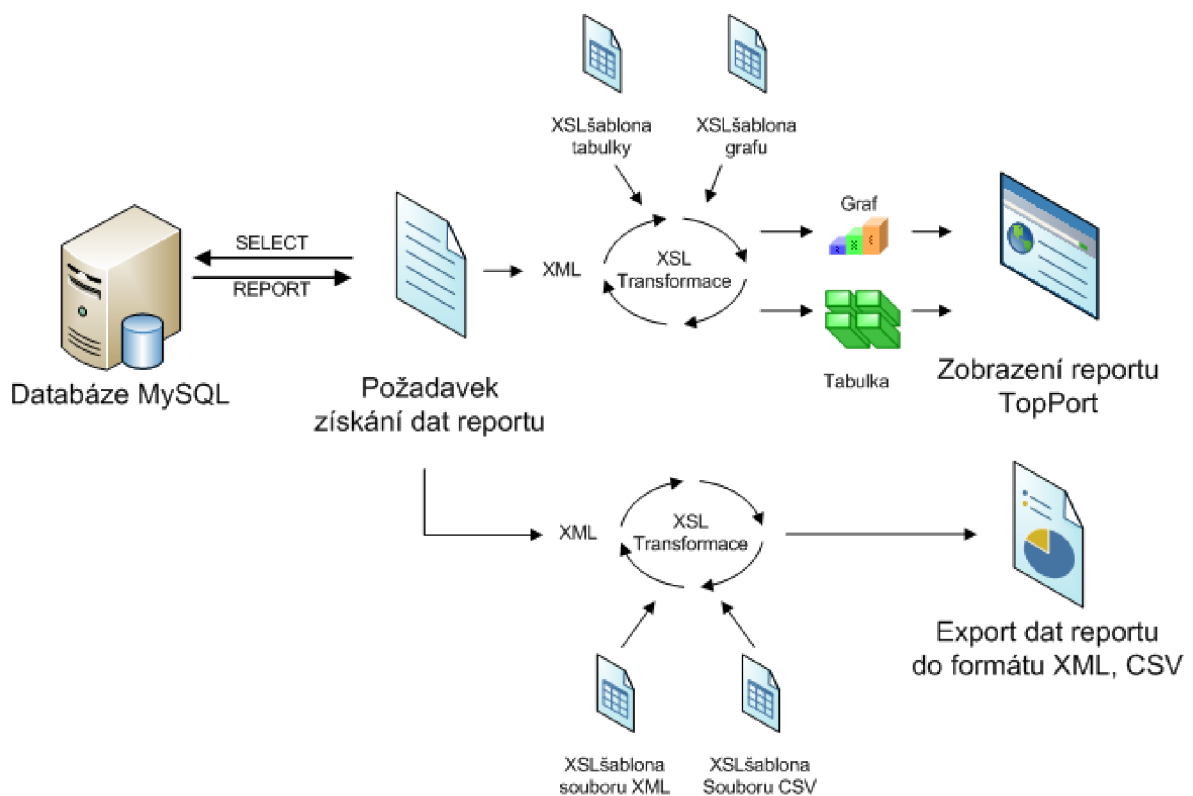
Obrázek 6 - Ilustrace zobrazení reportů
