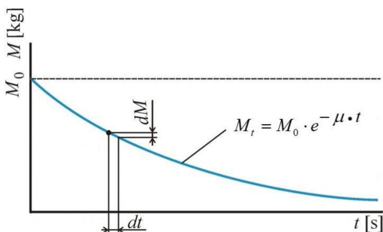
Obrázek 3 Grafické znázornění hmotnosti materiálu nad sítí v závislosti na čase [12]
