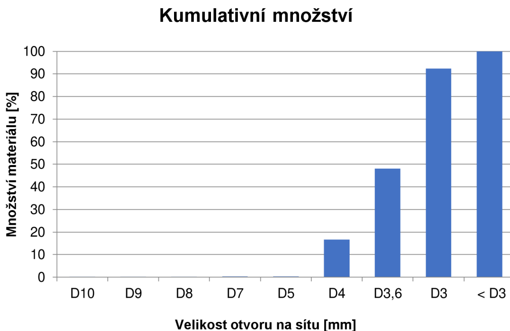
Obrázek 15 Kumulativní množství materiálu na sítích s obdélníkovými otvory
