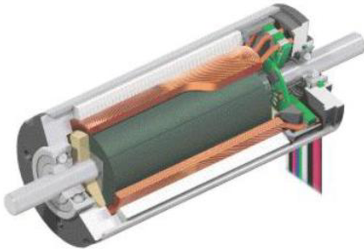
Obr.6. BLDC motor v řezu, převzato z [5]
