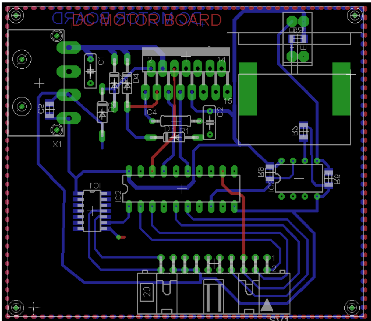
Obr.26. Deska plošného spoje modulu pro DC motor.
