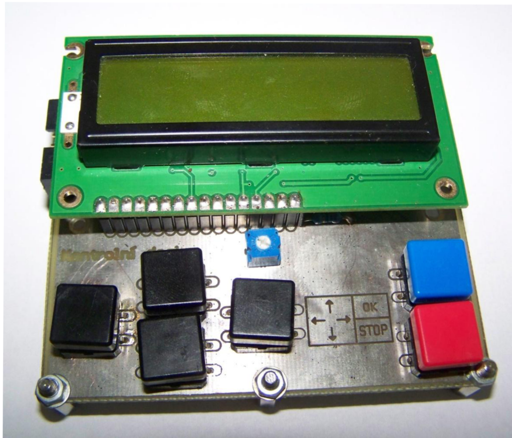
Obr.20. Řídící modul
