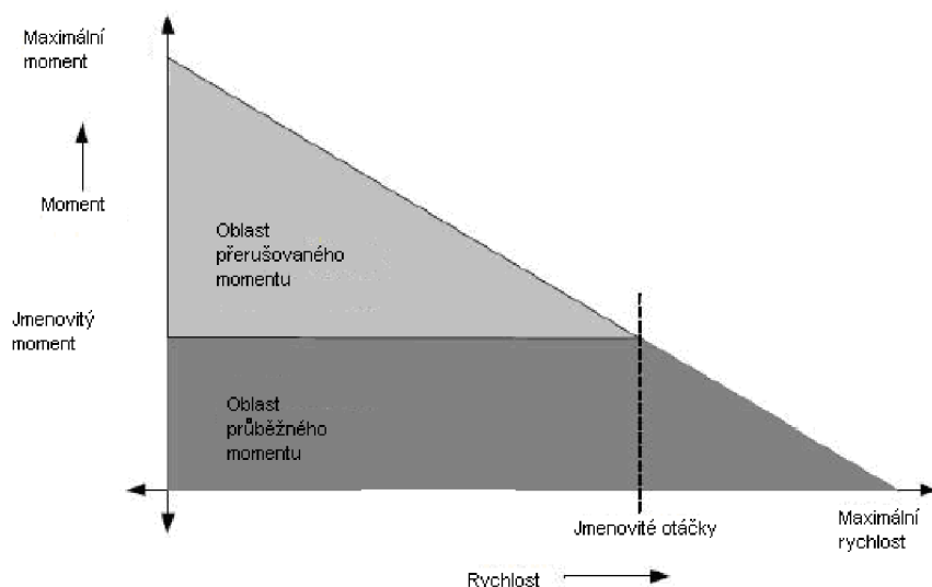
Obr.13. Charakteristika točivého momentu na rychlosti, převzato z[6]
