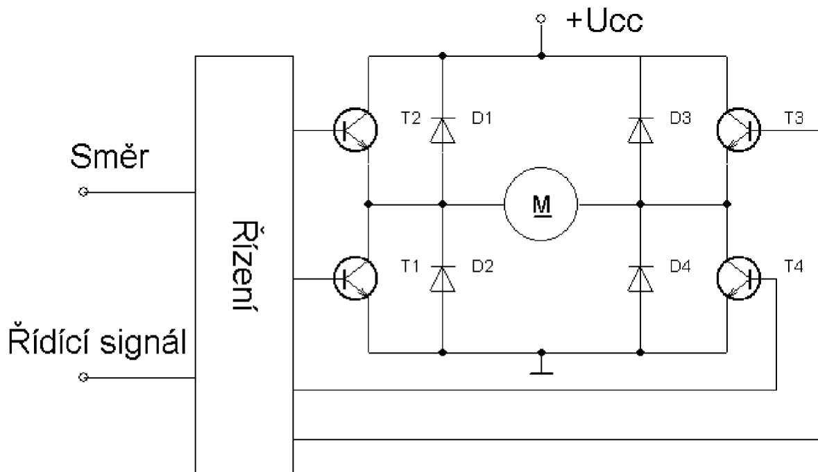
Obr.5. Čtyřkvadrantový budič
