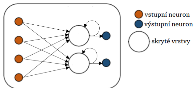
Obr. 16: Rekurentní neuronová síť [36]
