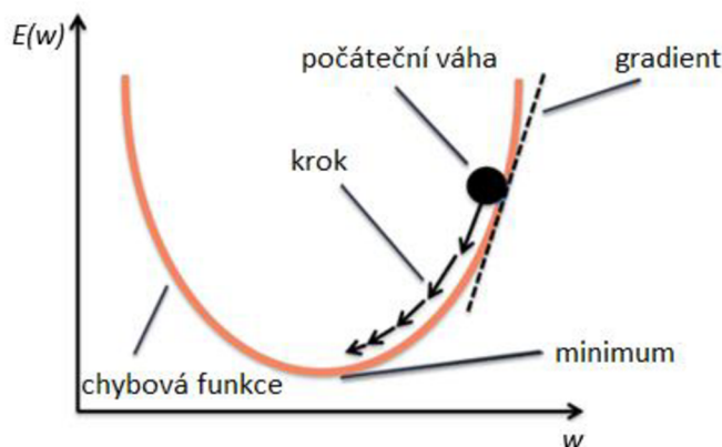
Obr. 18: Gradientní sestup [40]
