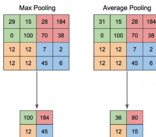
Obr. 21: Princip sdružování pro velikost okna 2 \times 2 px s hodnotou posunu 2 px [45]
