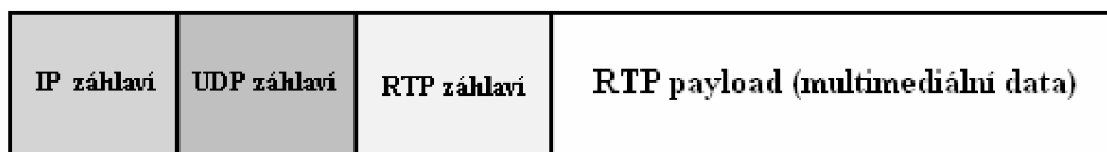
Obrázek 4.1: Datagram s paketem protokolu RTP
