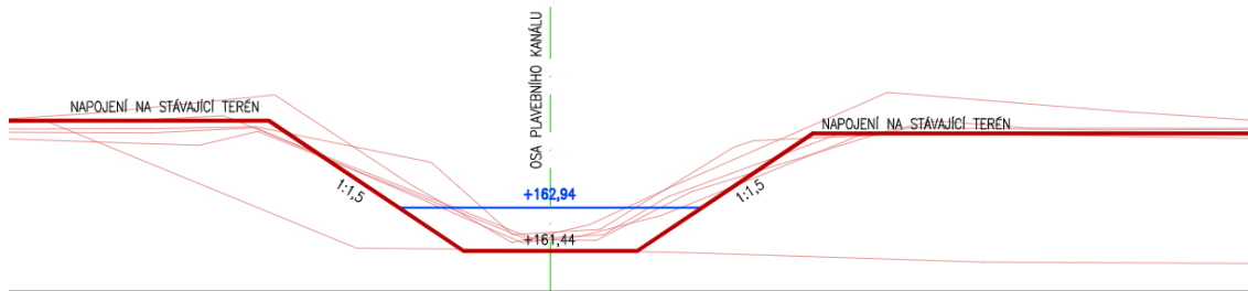
Obrázek 14 – Synoptické řezy PF 01 – 06
