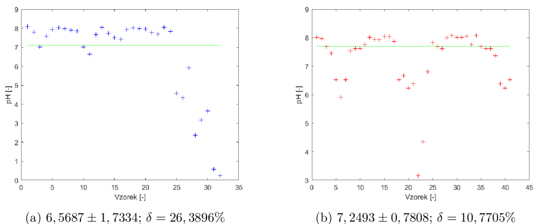
Obr. 8.1: Naměřené hodnoty pro pufrů o známé hodnotě pH, kde body jsou jednotlivé hodnoty a zelená linie značí deklarované pH pufru.
