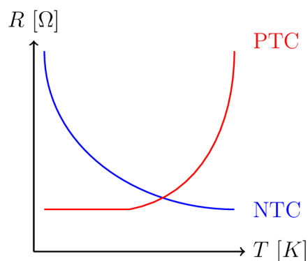
Obr. 3.4: Ilustrační znázornění závislosti termodynamické teploty T [K] a elektrického odporu R [\Omega] s pozitivním a negativním teplotním koeficientem.
