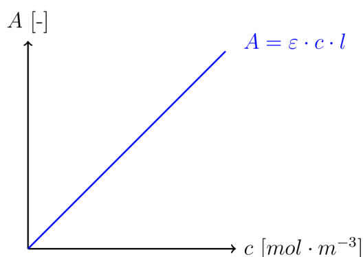
Obr. 2.2: Ilustrační znázornění závislosti absorbance A na molární koncentraci c [ \text{mol} \cdot \text{m}^{-3} ].
