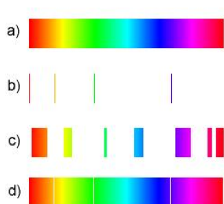
Obr. 1.3: Příklady druhů spekter – a) spojité spektrum, b) čárové (emisní) spektrum, c) pásové spektrum a d) absorpční čárové spektrum. [7]
