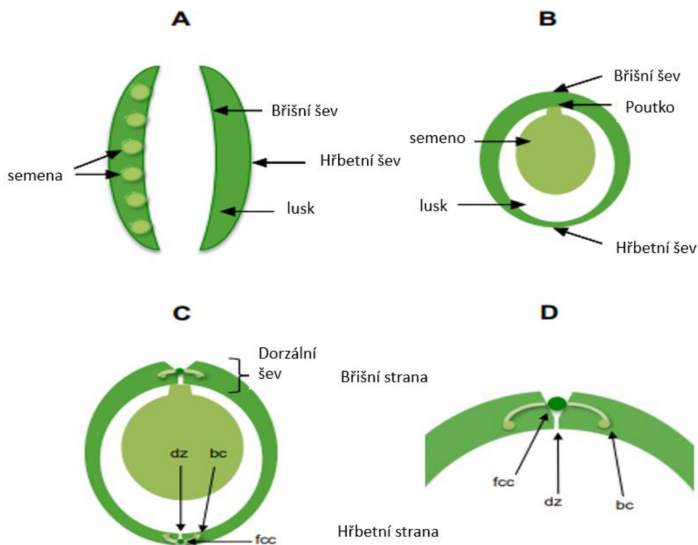
Obrázek 2: Struktura lusk u luskovin. (A) Průřez luskem, ve kterém jsou uzavřeny semena. (B) Průřez luskem, kde je semeno přichyceno skrz placentu ke švu. (C, D) Zvětšený pohled na průřez (převzato a upraveno z Ogutcen, 2018).
