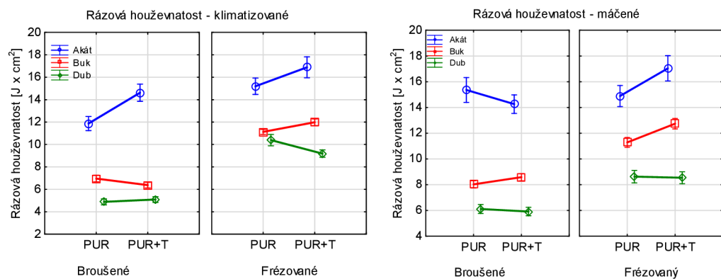
Obrázek 28 Analýza vlivu termosetů na rázovou houževnatost
