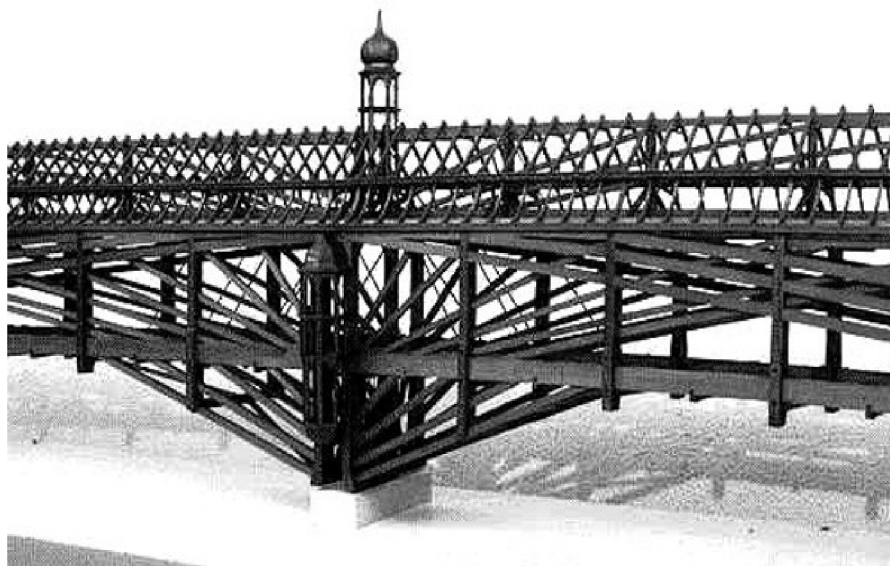
Obrázek 9 Model mostu z lepeného lamelového dřeva (Kuklík 2015)
