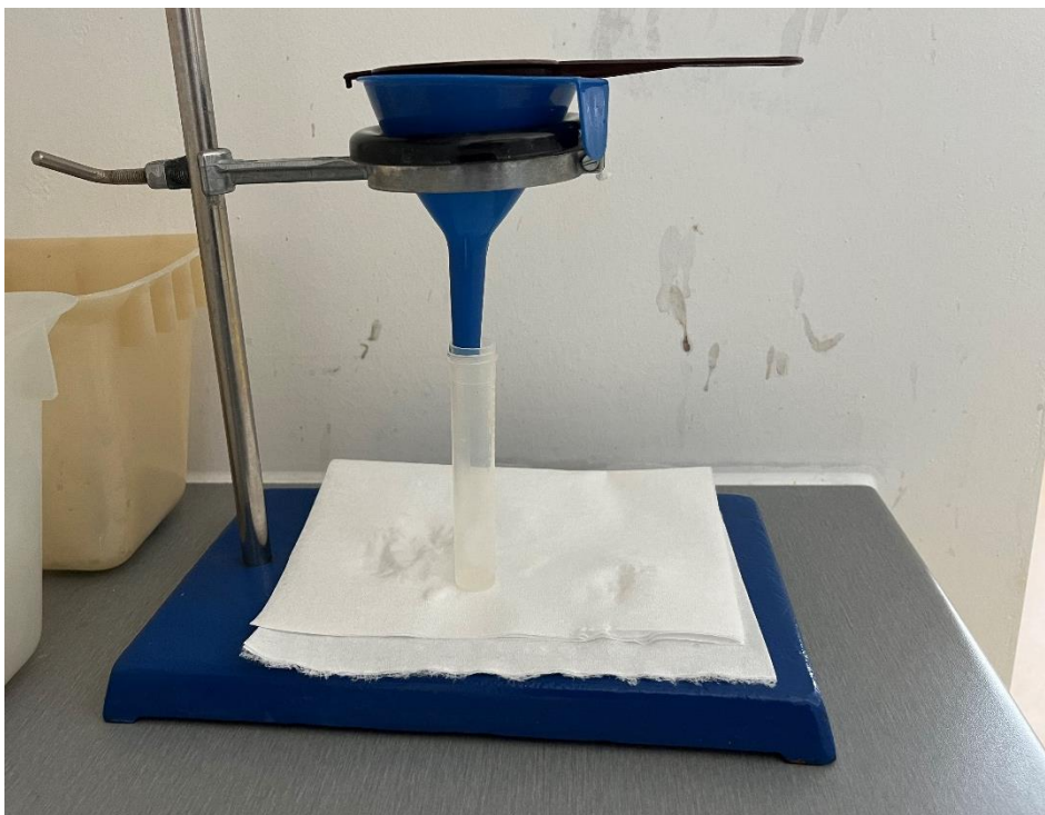
Obrázek 3.1: Flotační aparatura
