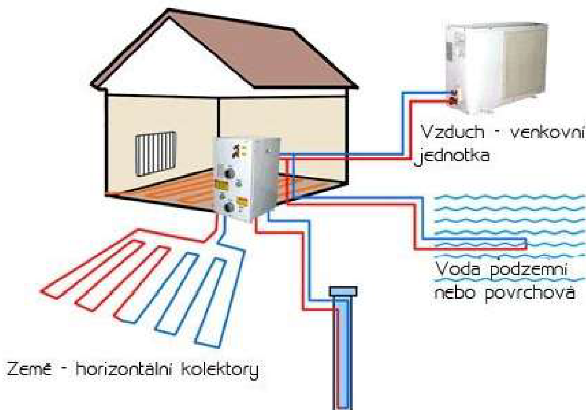
Obr. 2: Možnosti výroby tepla tepelným čerpadlem z nízkopotenciální energie [15]
