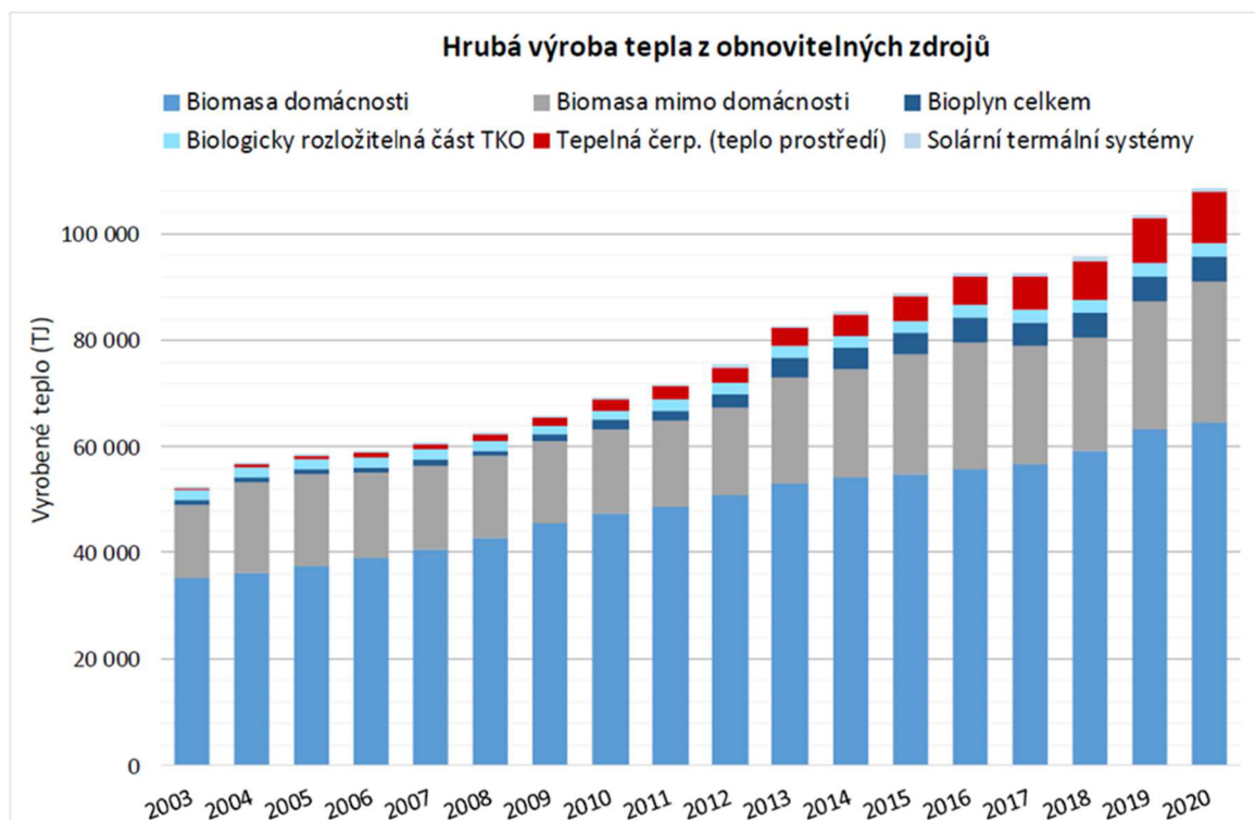
Obr. 1: Hrubá výroba tepla z obnovitelných zdrojů v ČR v letech 2003-2020 [11]
