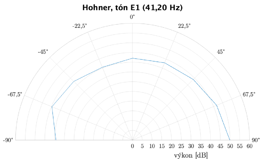
Obr. 3.58: Hohner – směrnost tónu E 1
