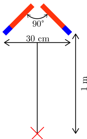
Obr. 4.13: Schéma rozestavení mikrofonů techniky NOS
