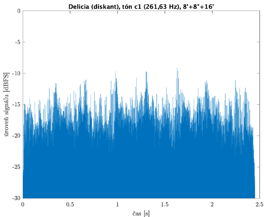
Obr. 3.9: Delicia – časový průběh tónu c^1 , 8'+8^\circ+16' rejstřík
