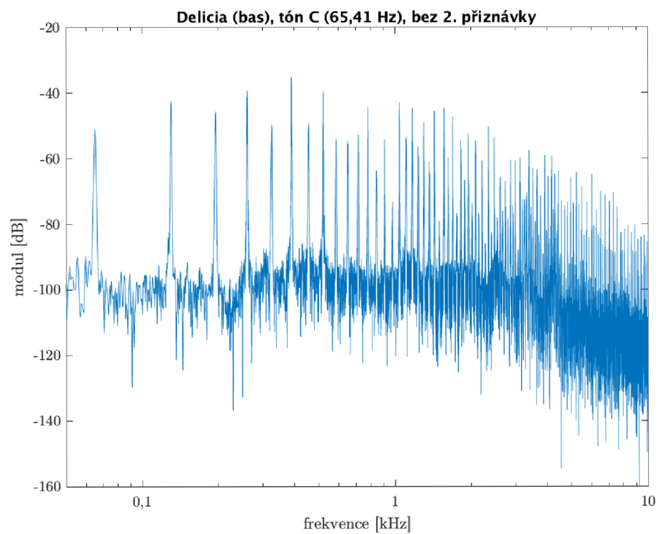
Obr. 3.13: Delicia – spektrum tónu C, bez 2. přiznávky
