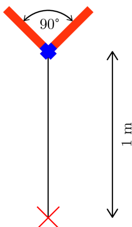
Obr. 4.1: Schéma rozestavení mikrofónů techniky XY
