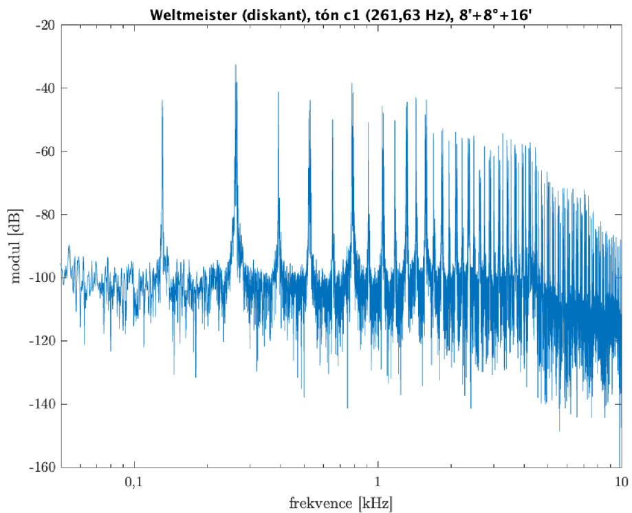
Obr. 3.18: Weltmeister – spektrum tónu c^1 , 8'+8^\circ+16' rejstřík
