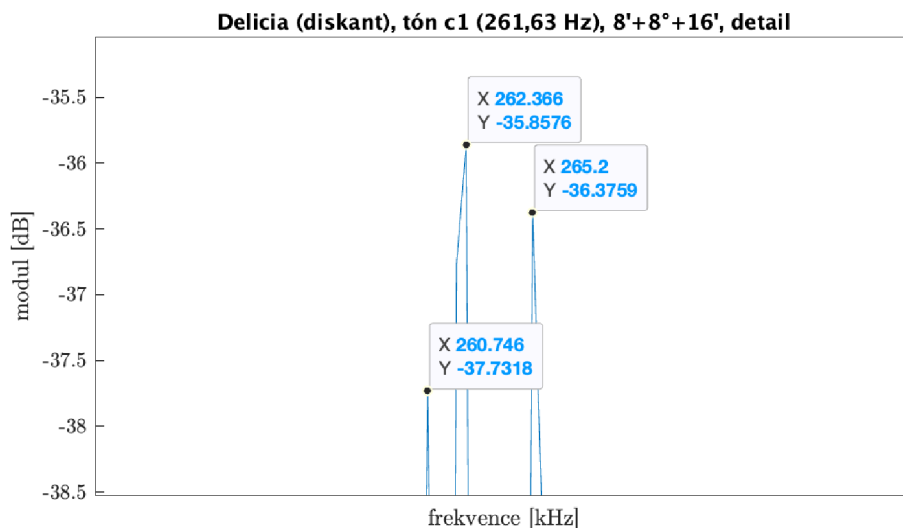
Obr. 3.8: Delicia – spektrum tónu c^1 , 8'+8^\circ+16' rejstřík, detailní pohled
