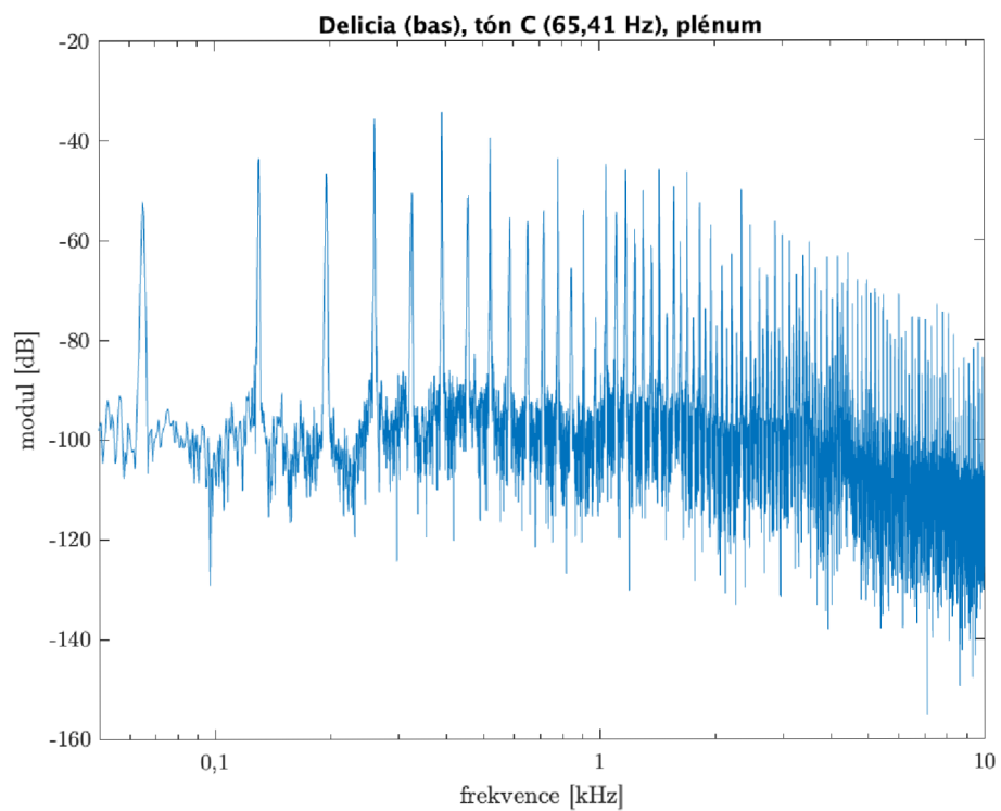
Obr. 3.12: Delicia – spektrum tónu C, plénium
