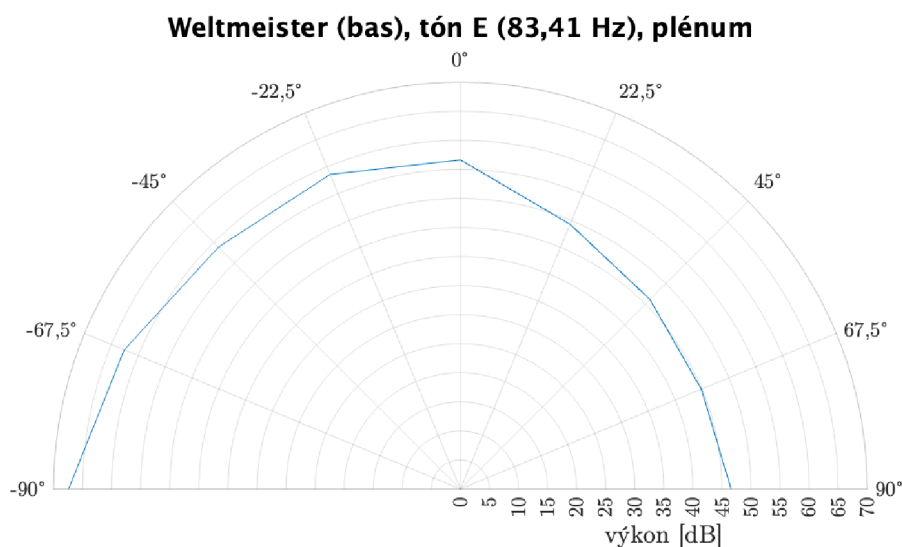
Obr. 3.53: Weltmeister – směrovost tónu E, plénium
