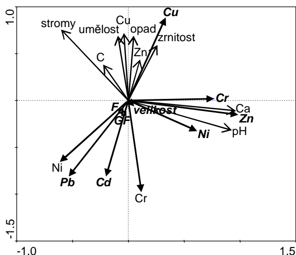
Obr. 22: RDA závislosti faktorů prostředí a populačních charakteristik P. scaber
