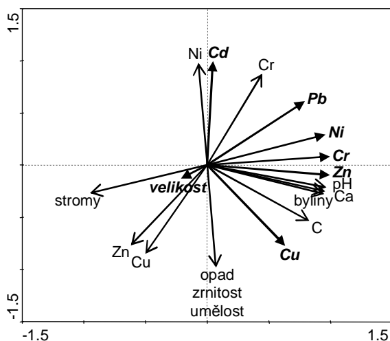
Obř. 21: RDA závislostí faktorů prostředí a populačních charakteristik P. collicola pozn. → faktory prostředí → charakteristiky stejnonožců
