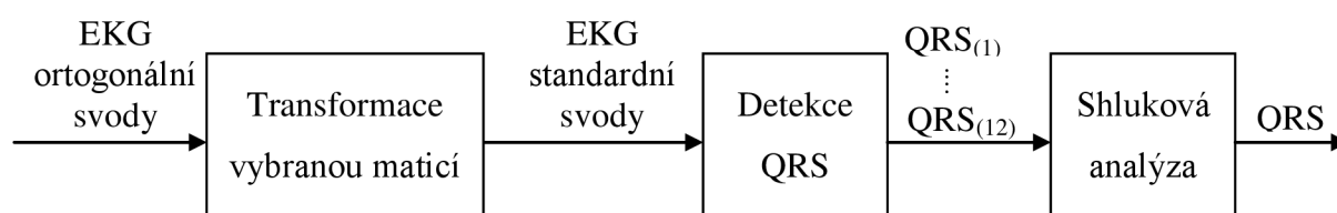
Obr. 4.1: Blokové schéma algoritmu pro detekci QRS komplexů v transformovaných svodech
