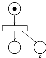
Obr. 3.3: Ukázkový proces.
