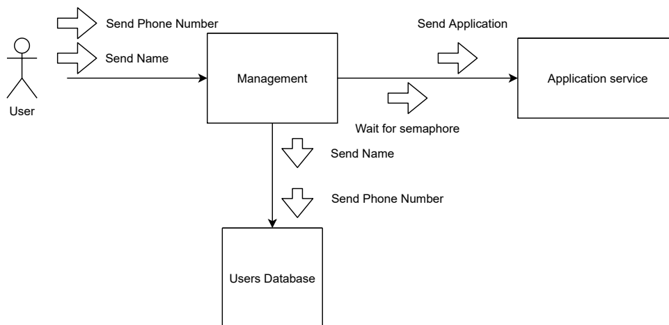
Obr. 2.4: Diagram spolupráce.
