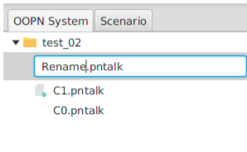
Obr. 6.7: Premenovanie súboru.
