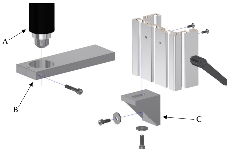
Obrázek 27: Držák měřáku
