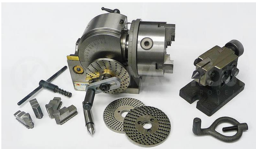
Obrázek 6: Dělicí přístroj s příslušenstvím BS-0-J, TOS UIG 125/3 - 2 [7]
