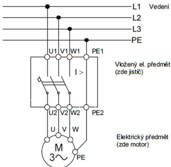
Obr. 1.1 Příklad označení vodičů a svorek elektrických předmětů ve schématu
