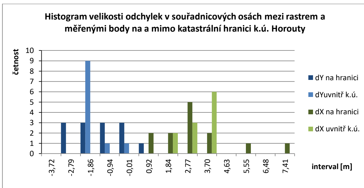
Obr. 30 Histogram velikosti odchylek v souřadnicových osách mezi rastrem a měřnými body na a mimo katastrální hranici k.ú. Horouty
