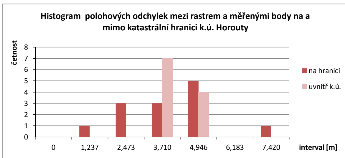
Obr. 29 Histogram polohových odchylek mezi rastrem a měřnými body na a mimo katastrální hranici k.ú. Horouty
