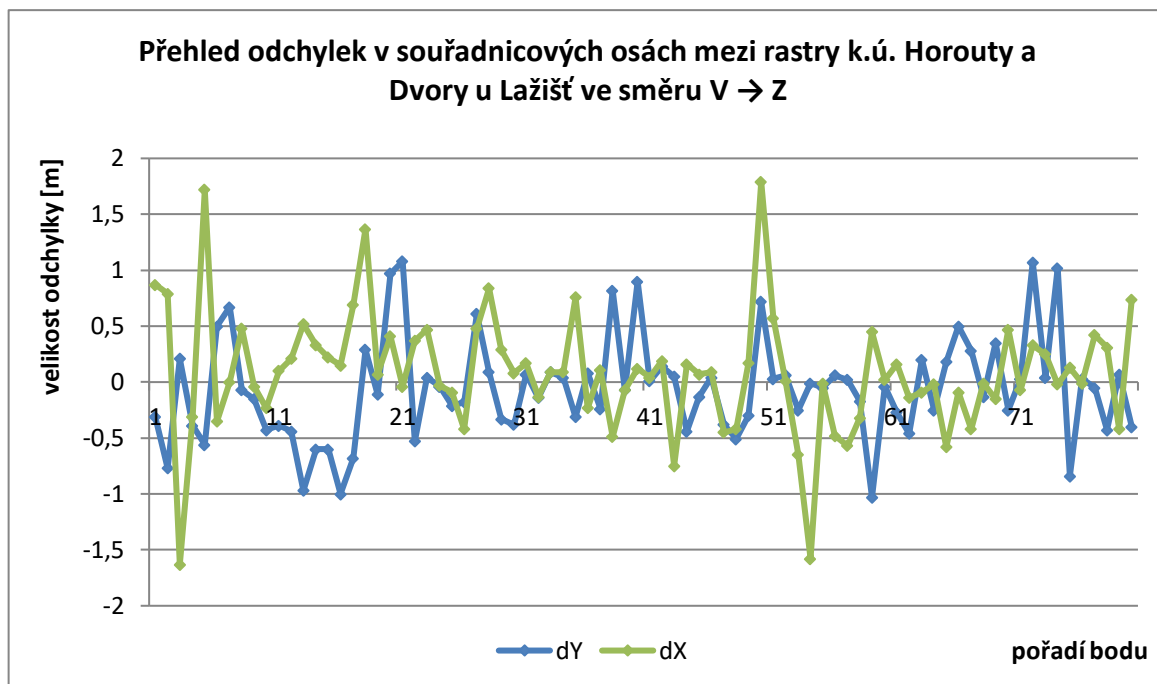
Obr. 28 Přehled odchylek v souřadnicových osách mezi rastry k.ú. Horouty a Dvory u Lažišť ve směru V → Z
