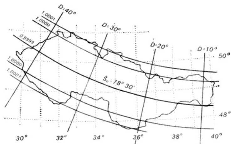
Obr. 4 Průběh délkového zkreslení Křovákova zobrazení [6]
