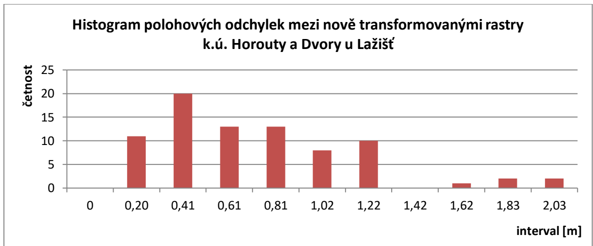
Obr. 33 Histogram polohových odchylek mezi nově transformovanými rastry k.ú. Horouty a Dvory u Lažišť
