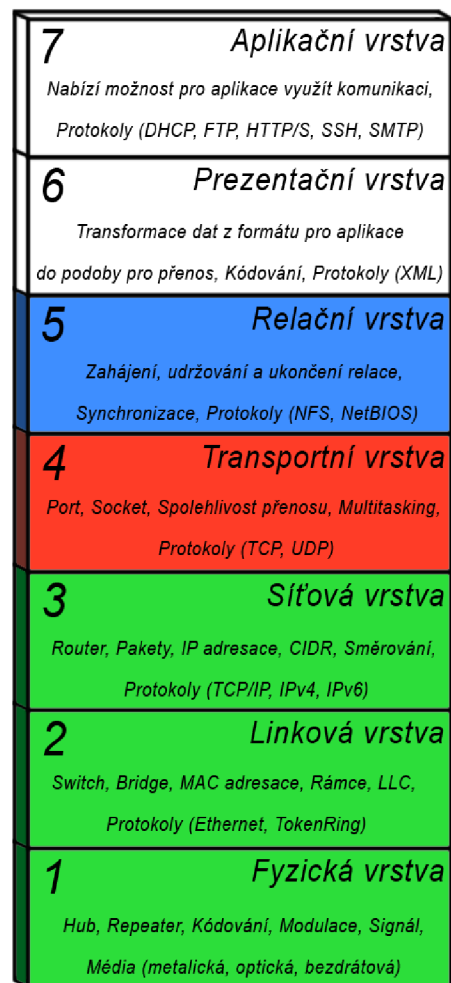
Obrázek 4-5 transportní vrstva. Zdroj: vlastní
