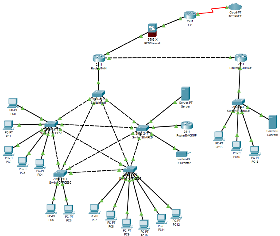
Obrázek 6-1 REDSoftware model
