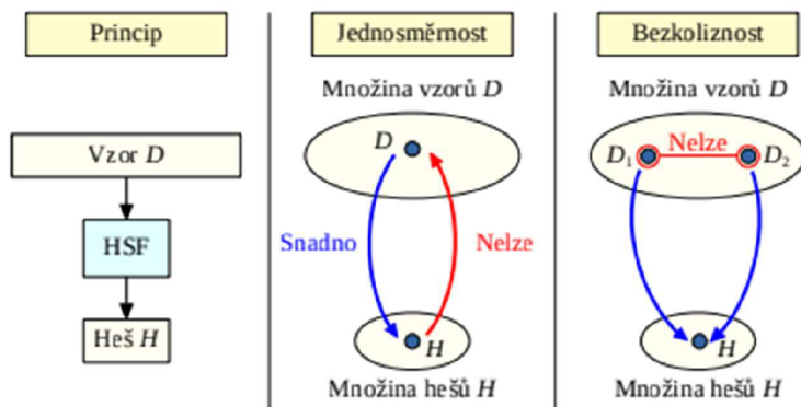
Obrázek 8 Hashovací funkce Zdroj: [8]
