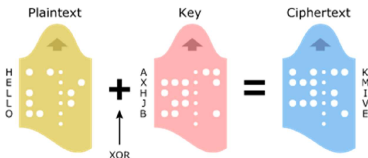
Obrázek 7 Vernamova šifra
