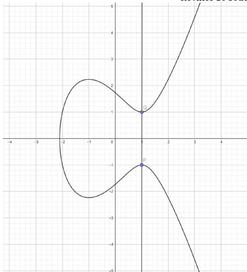
Obrázek 4 Sčítání bodů druhý příklad, součet v bodu O
