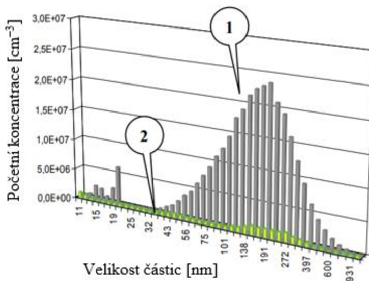
Obrázek 12 Velikostní distribuce částic v ustálené fázi spalování dřevěných polen. 1) vypnutý EO 2) zapnutý EO. Převzato z [17].
