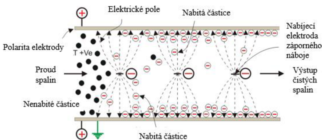
Obrázek 7 Princip elektrostatičké odlučovače. Převzato z [27].
