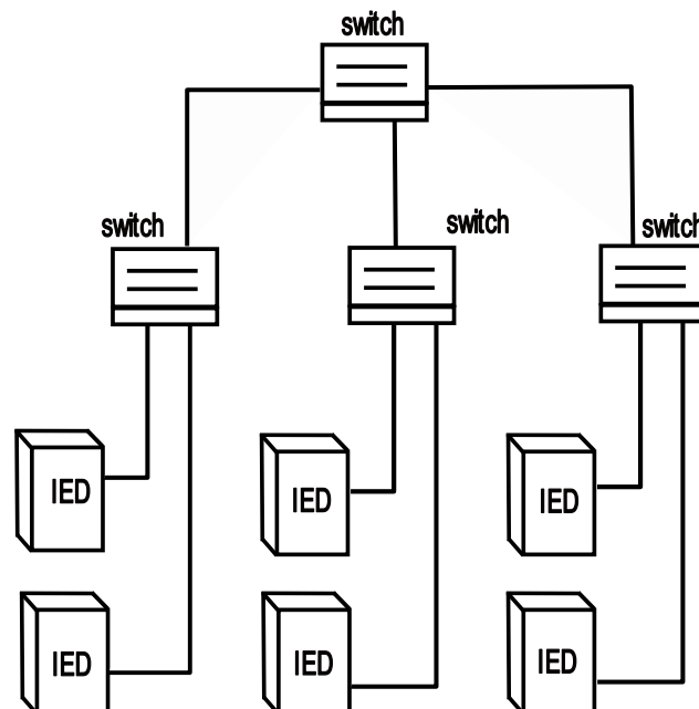
Obrázek 2.11 Topologie hvězda
