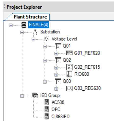
Obrázek 7.2 Struktura projektu
