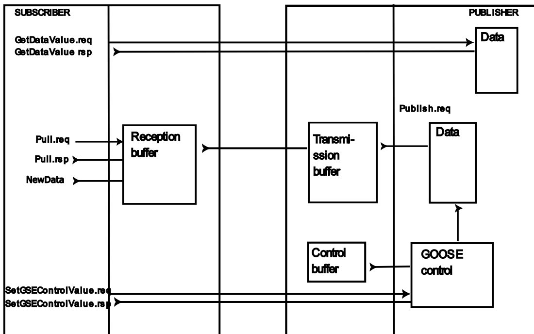
Obrázek 2.5 Vydavatel/Odběratel komunikace
