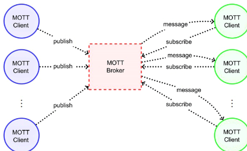
Obrázek 6.1 MQTT [20]
