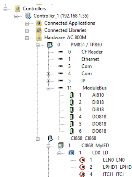
Obrázek 7.8 Hardware struktura
