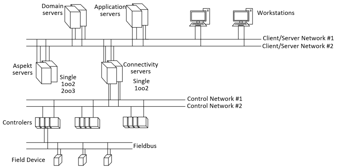
Obrázek 3.3 Topologie DCS
