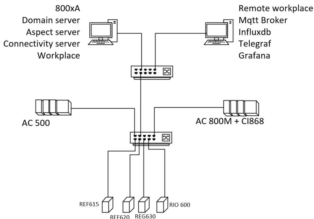
Obrázek 7.1 Topologie sítě
