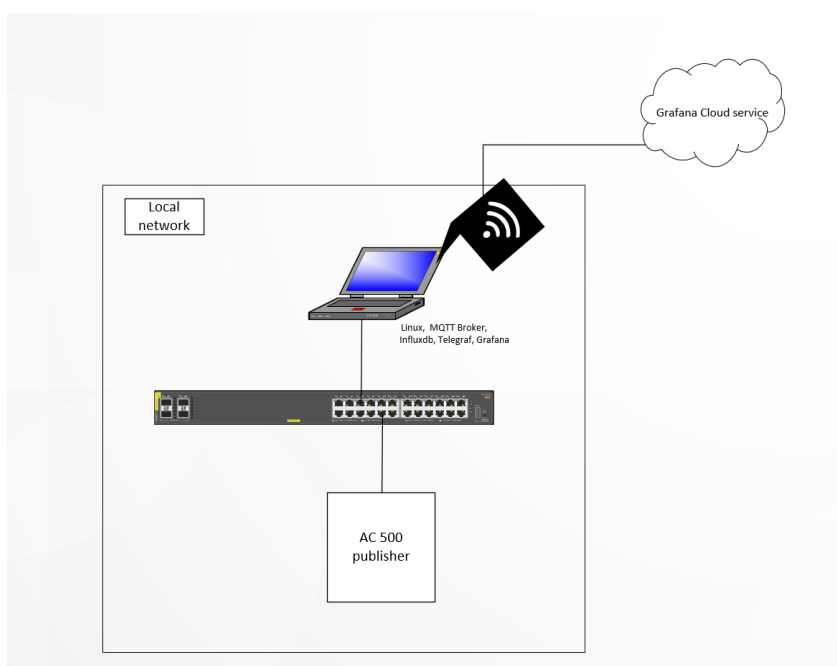
Obrázek 7.19 Zapojení aplikace
