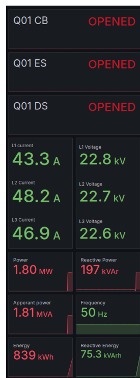
Obrázek 7.24 Testování REF620
