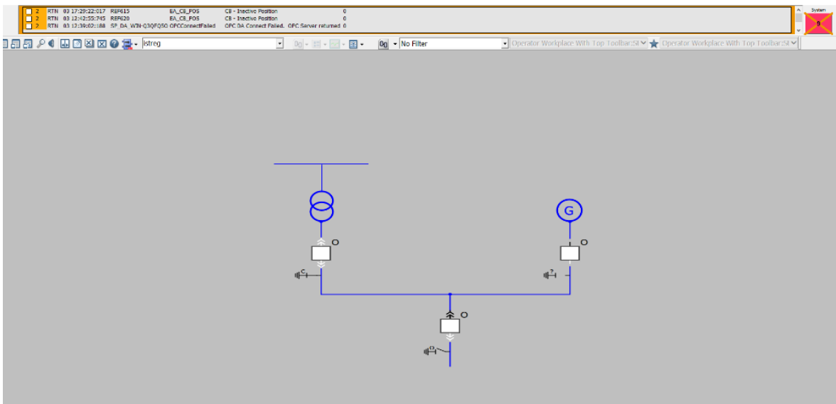
Obrázek 7.18 SLD
