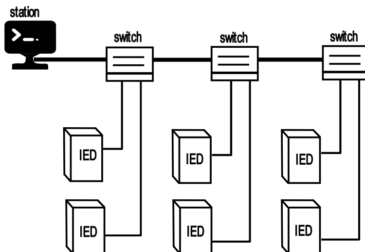
Obrázek 2.9 Topologie sběrnice
