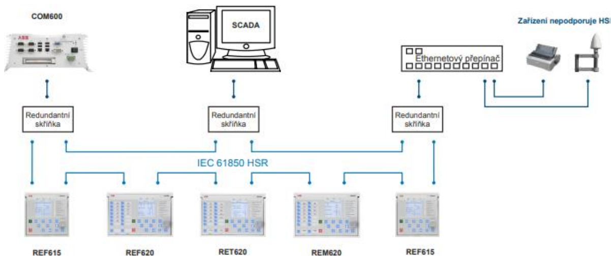
Obrázek 2.13 HSR protokol [12]
