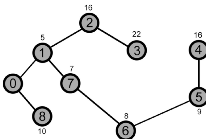
Obr. 12: Výsledné nejkratší cesty k uzlům
