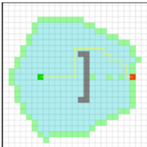
Obr. 16: Výsledek při zavedení Chebyschevovy vzdálenosti [5]
