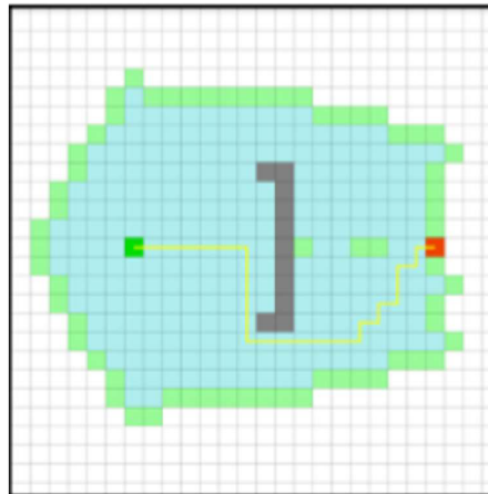
Obr. 14: Výsledek při zavedení Euklidovské heuristiky [5]
