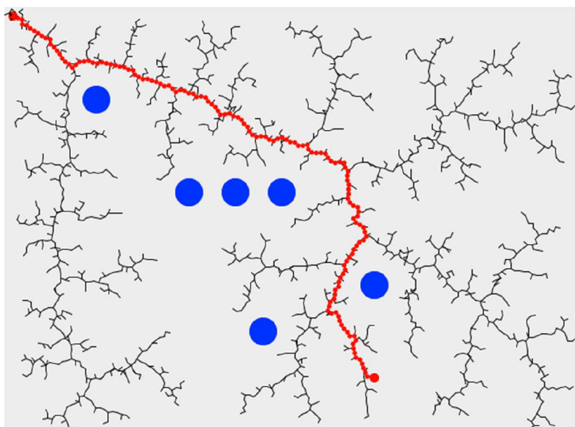
Obr. 10: Výsledek algoritmu RRT [12]
