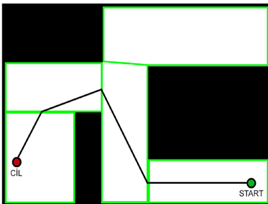
Obr. 17: Výsledná cesta s optimalizací NavMesh
