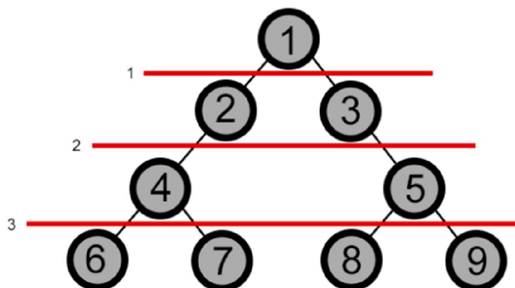
Obr. 9: Schéma prohledávání do šířky
