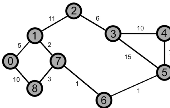
Obr. 11: Graf uzlů s cenami přechodů
