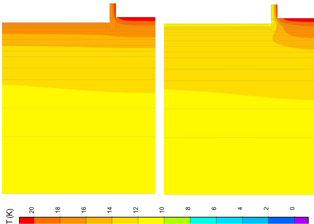
Obrázek 14-5: Detail 01_00 – A1 - rozložení teplot září a říjen
