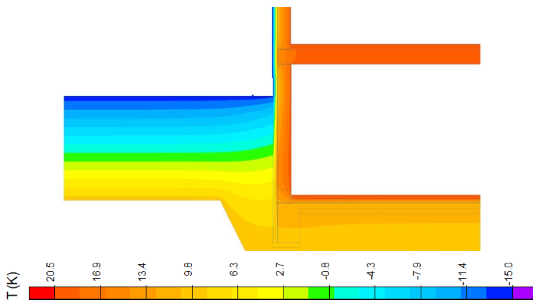
Obrázek 14-35: Detail 05_00 – E1 rozložení teplot
