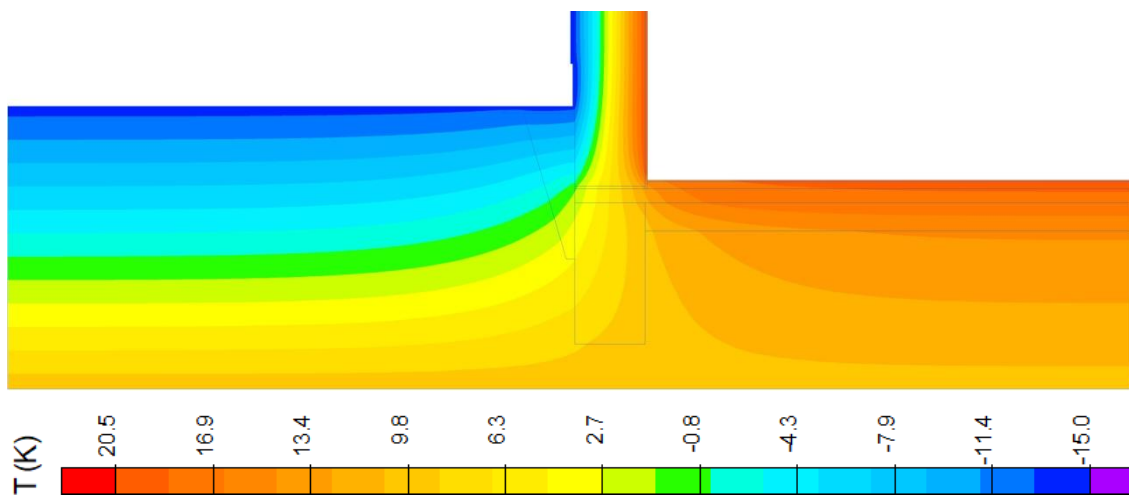
Obrázek 14-23: Detail 03_00 – E1 rozložení teplot
