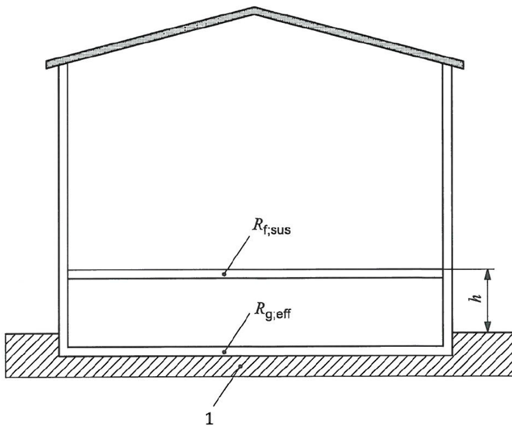
Obrázek 8-2: Schéma zvýšené podlahy [3]
