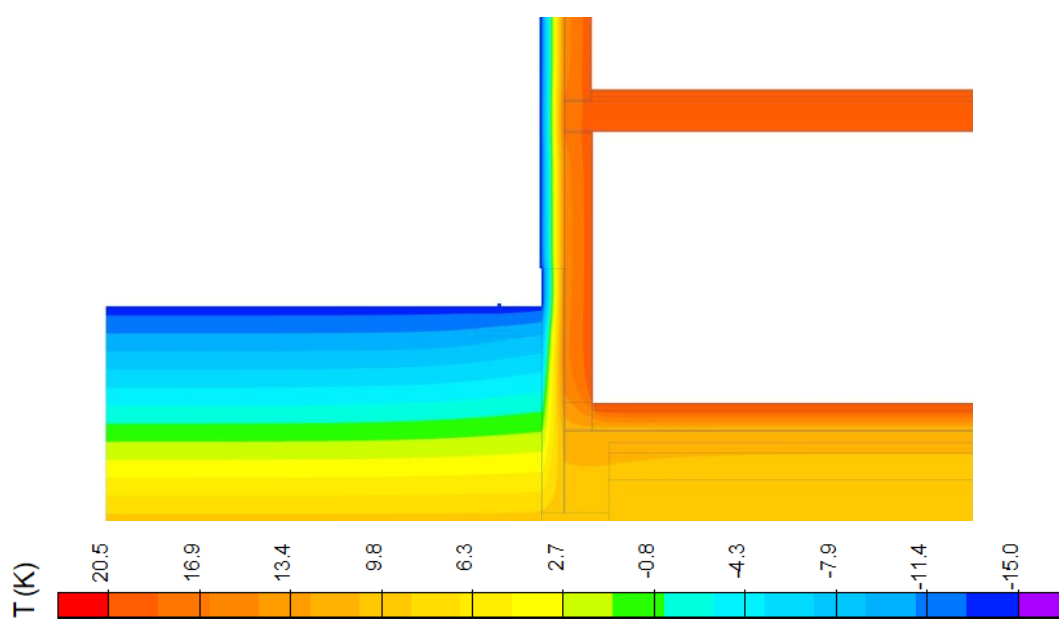
Obrázek 14-33: Detail 04_02 – E1 rozložení teplot
