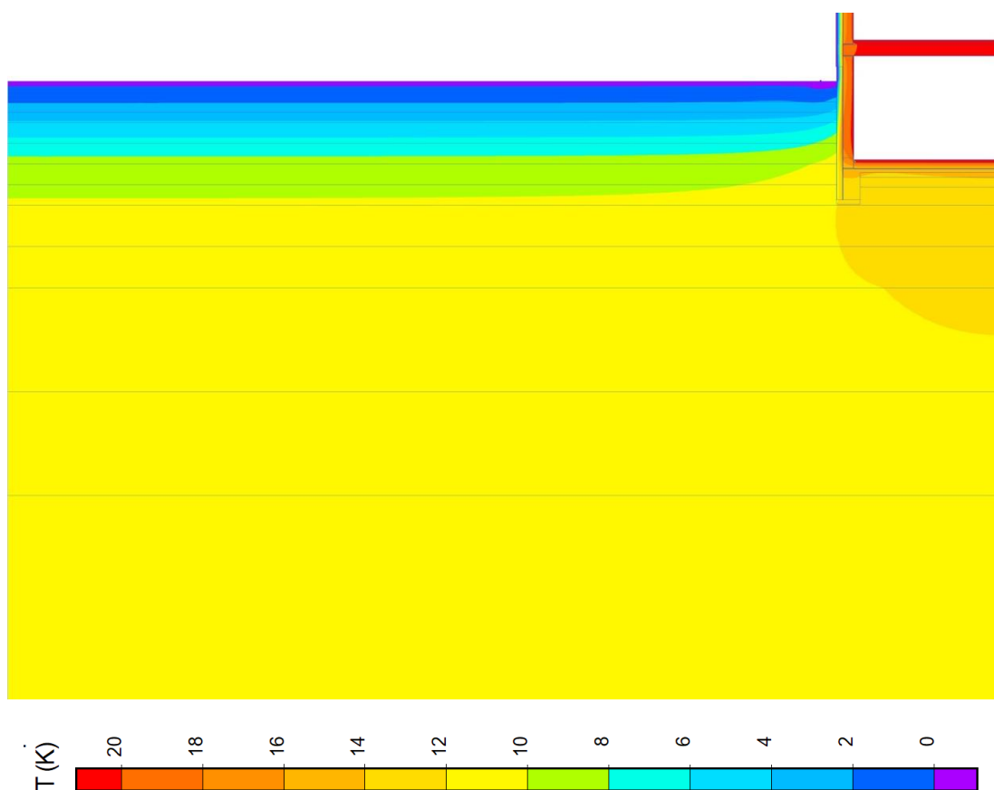
Obrázek 14-36: Detail 05_01 – A1 rozložení teplot leden
