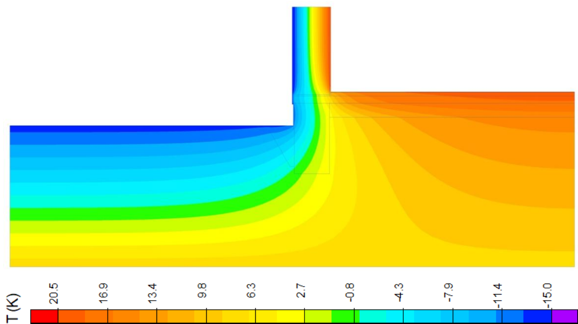
Obrázek 14-10: Detail 01_00 – D1 rozložení teplot
