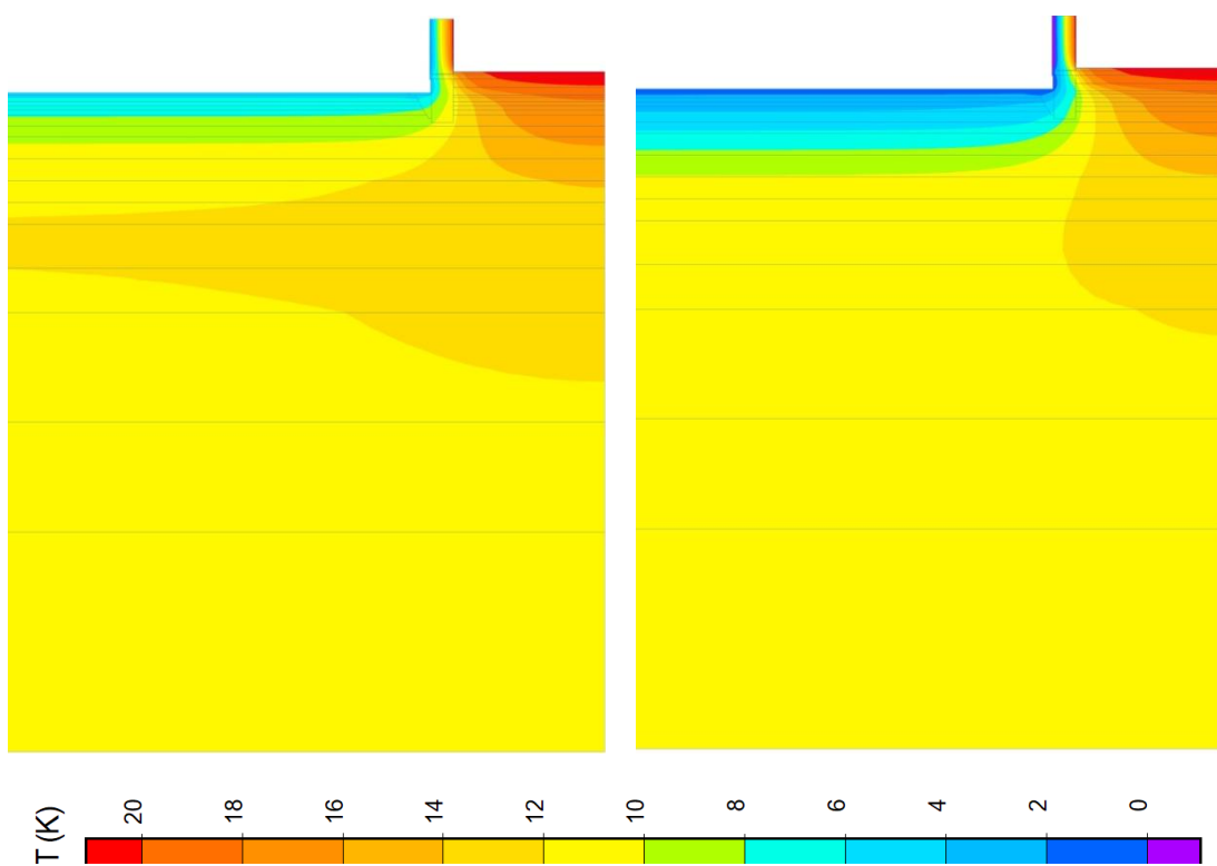
Obrázek 14-6: Detail 01_00 – A1 - rozložení teplot listopad a prosinec
