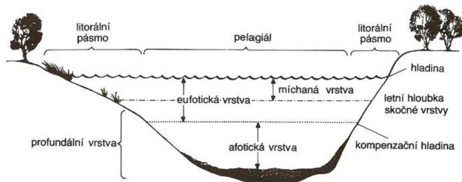
Obr. 7: Schéma horizontálního a vertikálního členění vodní nádrže (Lellák a Kubíček, 1992).
