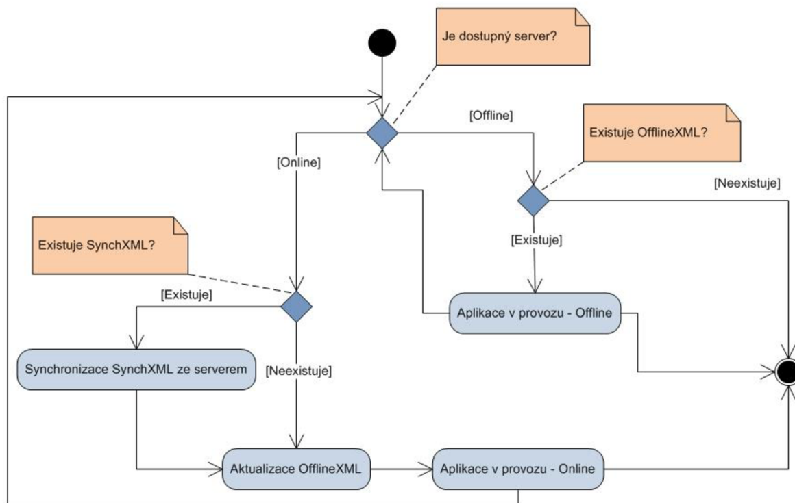
Obrázek 6.5: Proces zavádění lokální aplikace.
