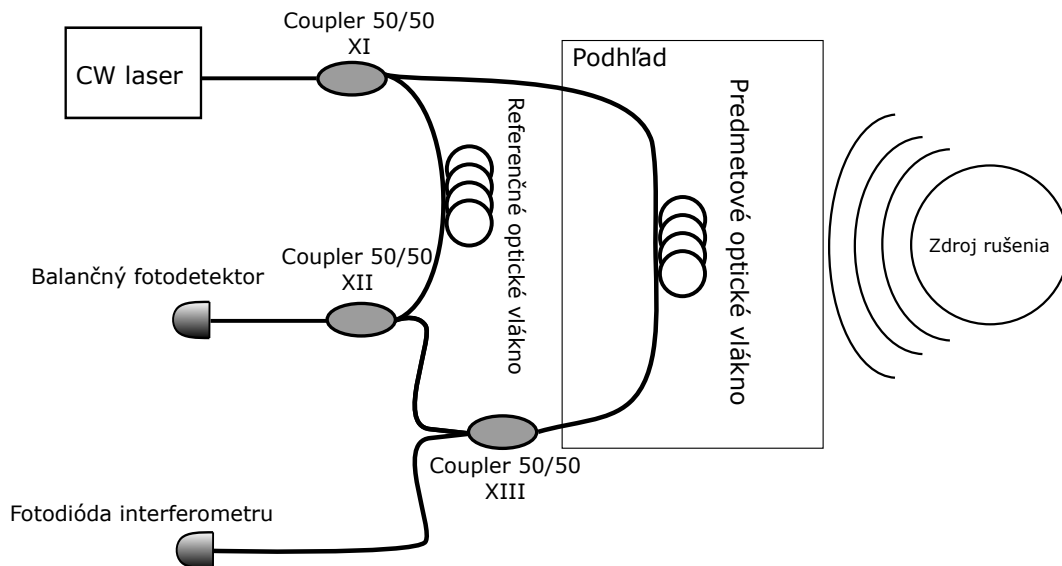
Obr. 2.1: Schéma zapojenia pracoviska pre nedátový prenos s využitím vláknového MZI
