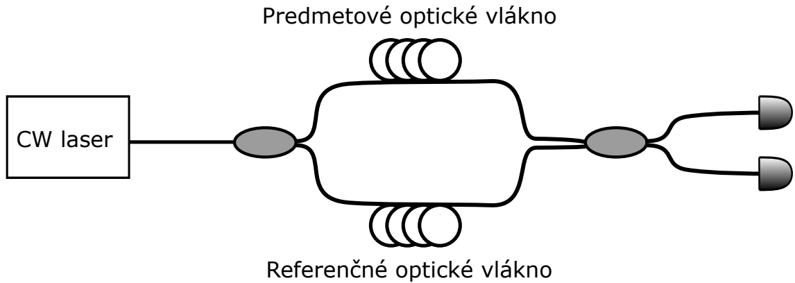
Obr. 1.9: Vlákňový Mach-Zehnderov interferometer
