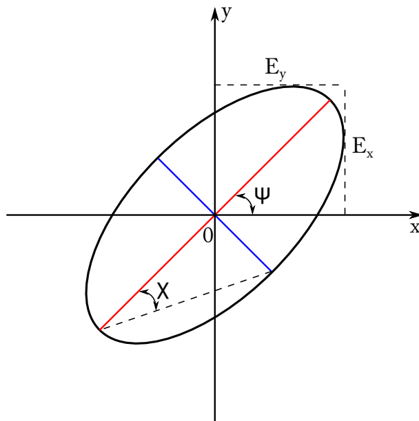
Obr. 1.2: Polarizačná elipsa
