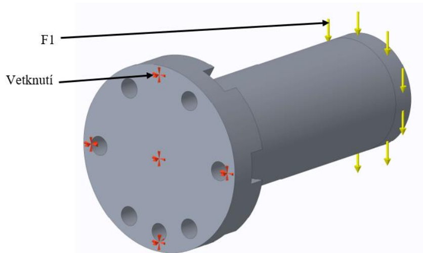
Obrázek 35: Výpočtový model připojovací příruby
