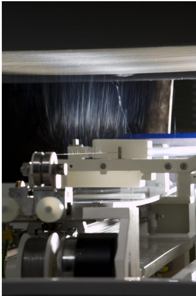
Obrázek 4: Zvlákňování technologií Nanospider [12]
