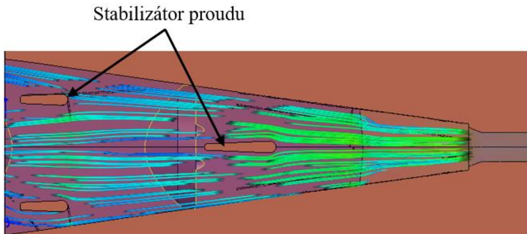
Obrázek 31: Simulace proudění vzduchu okolo příček
