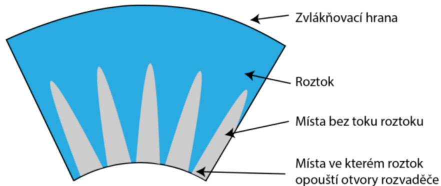
Obrázek 21: Schéma rozptýlení polymeru po ploše zvlákňovacího kužele [24]
