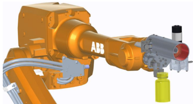
Obrázek 39: Robot IRB 2600 TYPE C se zvlákňovací jednotkou
