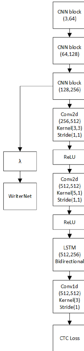
Obrázek 3.4: Schéma multi-task sítě
